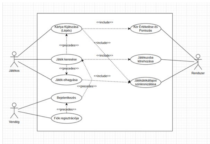
3.1. ábra. Előzetes használatieset-diagram Az ábra a draw.io [1] alkalmazás segítségével készült.
