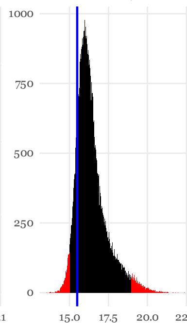
Decile 9
