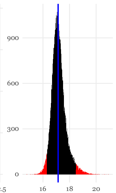
Decile 10
