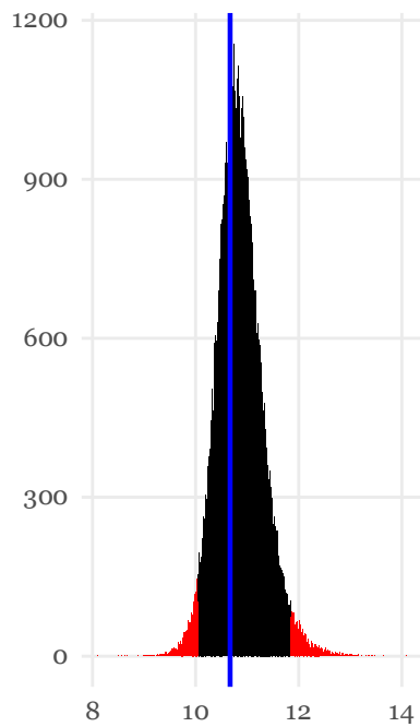
Decile 8
