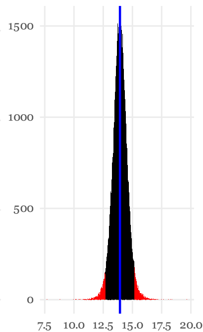
Decile 10
