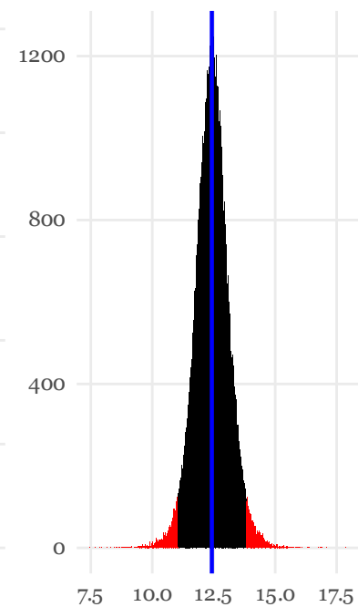
Decile 9
