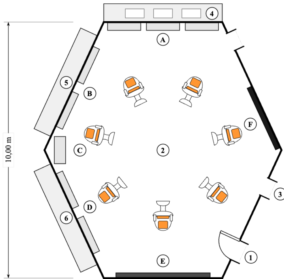
Abbildung 5: Aufbau des Operationsraums
