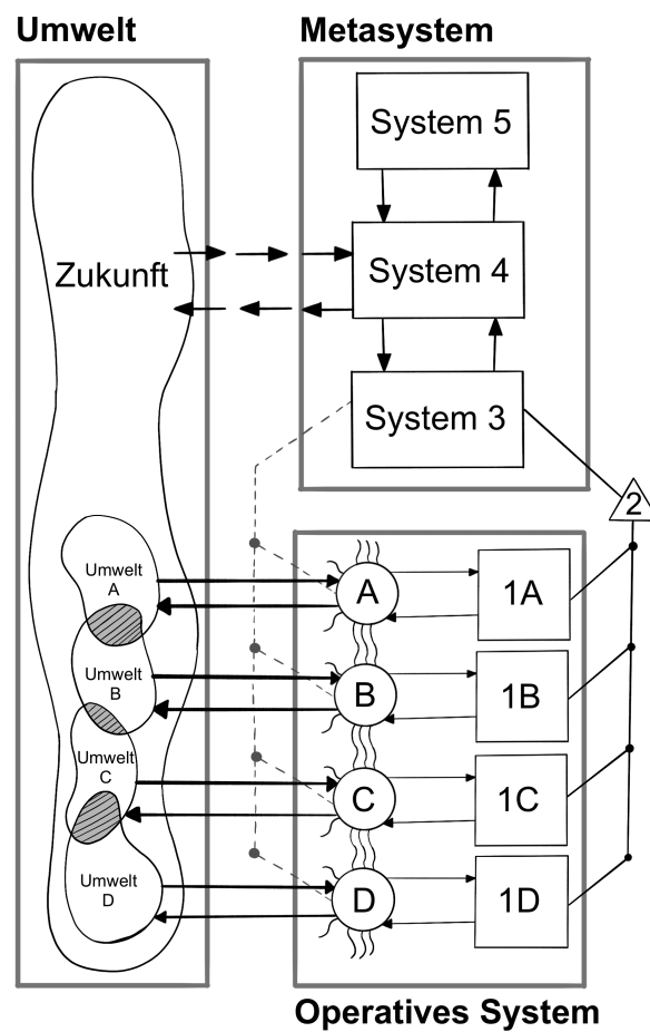
Abbildung 1: Aufbau des Viable System Model
