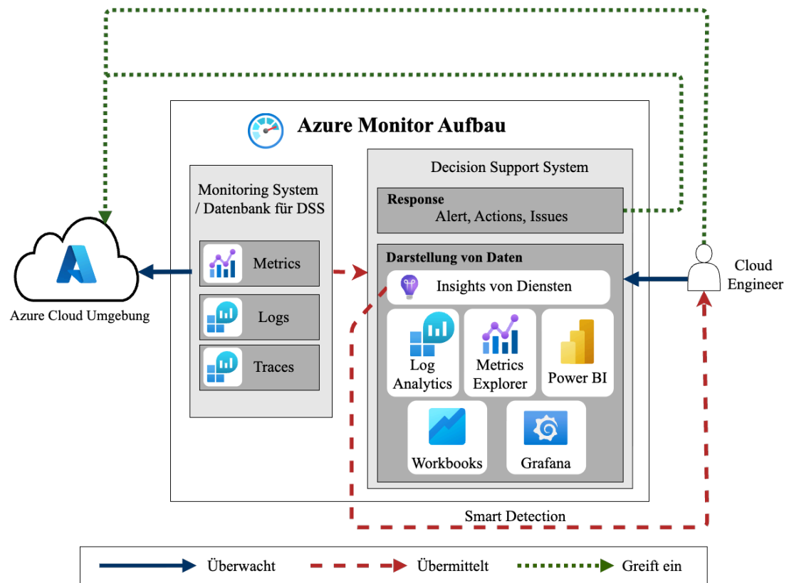
Abbildung 9: Architektur von Azure Monitor
