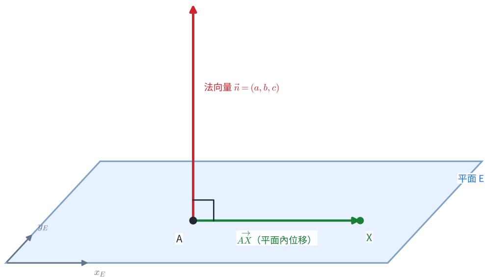
圖 1 | 平面內的每一個位移都與法向量垂直；這個內積條件就是點法式。
