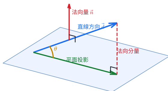
圖 10 | 直線在法向量上的投影決定離開平面的程度，因此線面角使用正弦。
