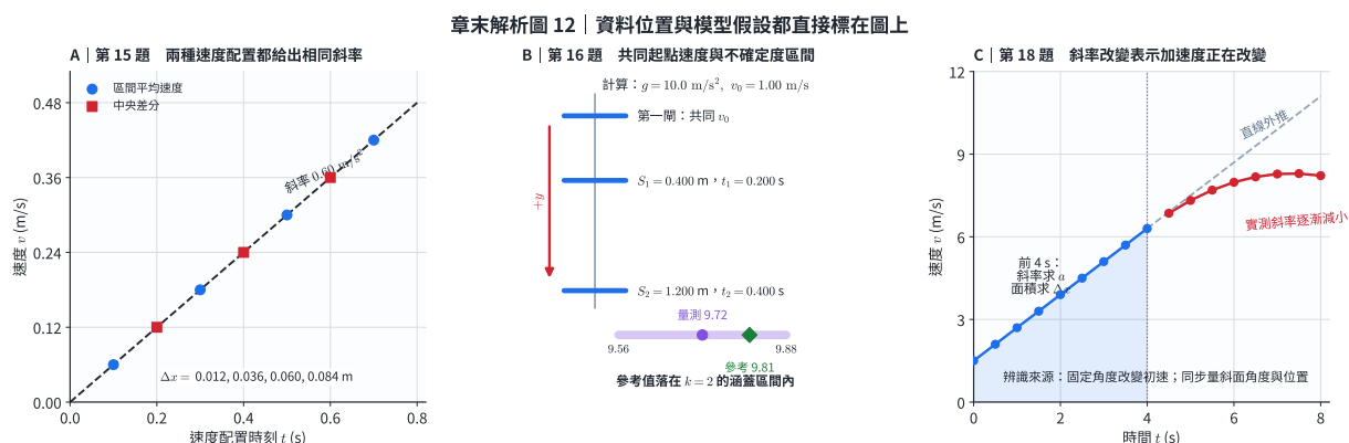
圖 12 | 章末解析第 15、16、18 題：A 比較區間平均與中央差分速度；B 以固定第一開建立共同 v_0 ，並畫出 k = 2 的涵蓋區間；C 比較前段直線模型、後段彎曲資料與線性外推。
