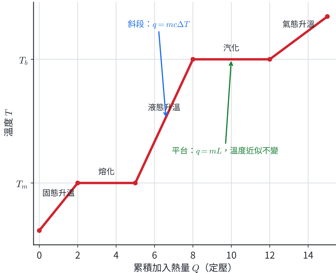
純物質在定壓下的加熱曲線
