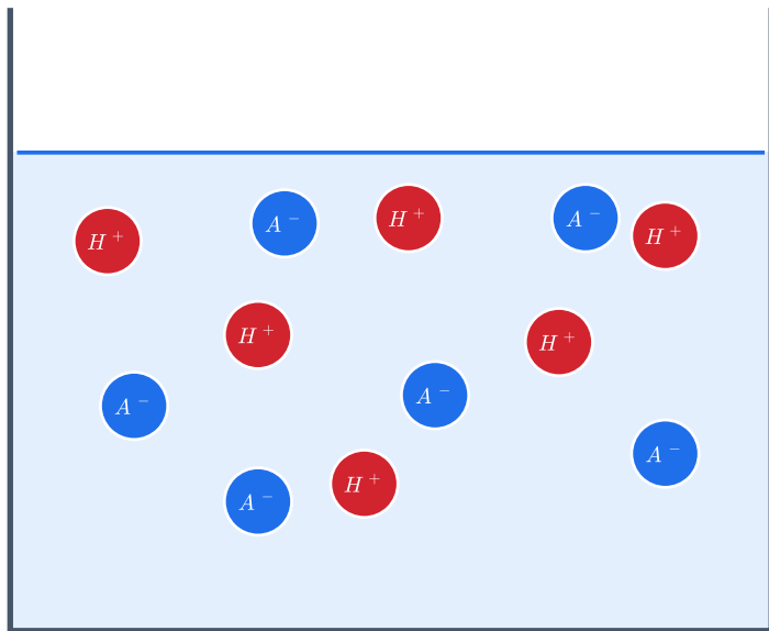
強酸 HA：近乎完全游離
