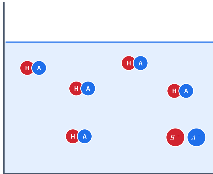
弱酸 HA：只有一部分游離
