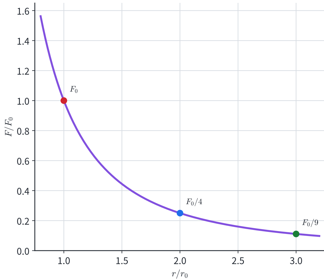
質量固定時的平方反比
