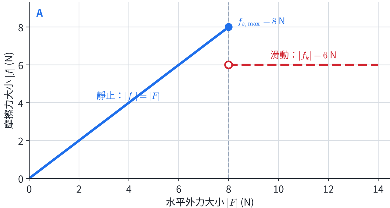
摩擦力大小隨外力改變
