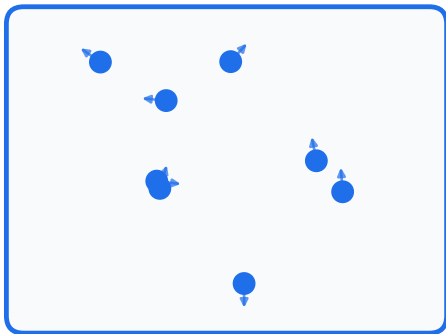
同為 8 個粒子：較低溫
