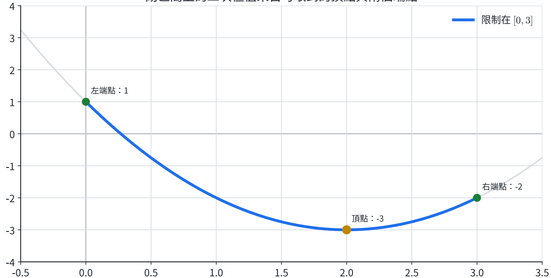
閉區間上的二次極值來自可取到的頂點與兩個端點
