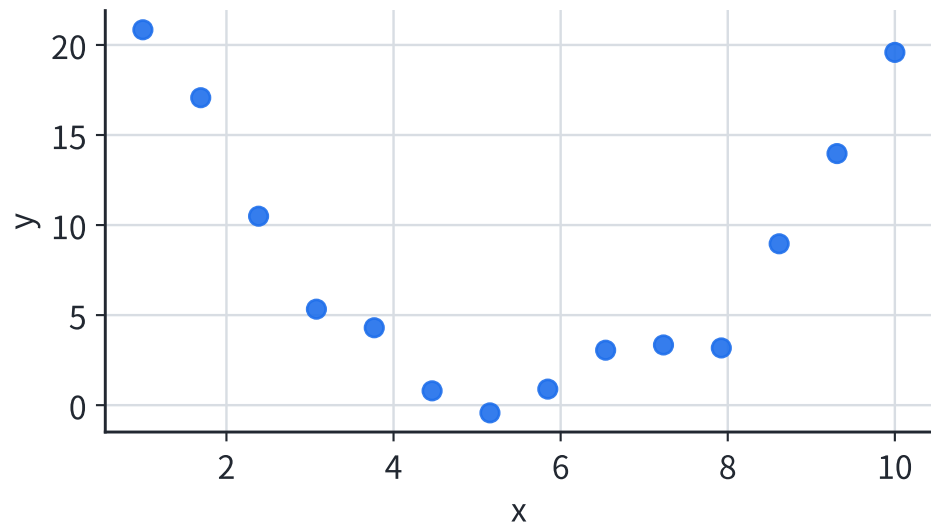
曲線關係； r 接近 0 ( r=-0.10 )
