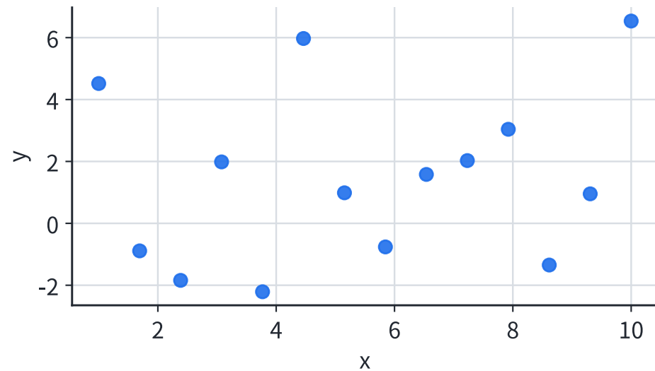
線性相關接近 0 ( r=0.21 )
