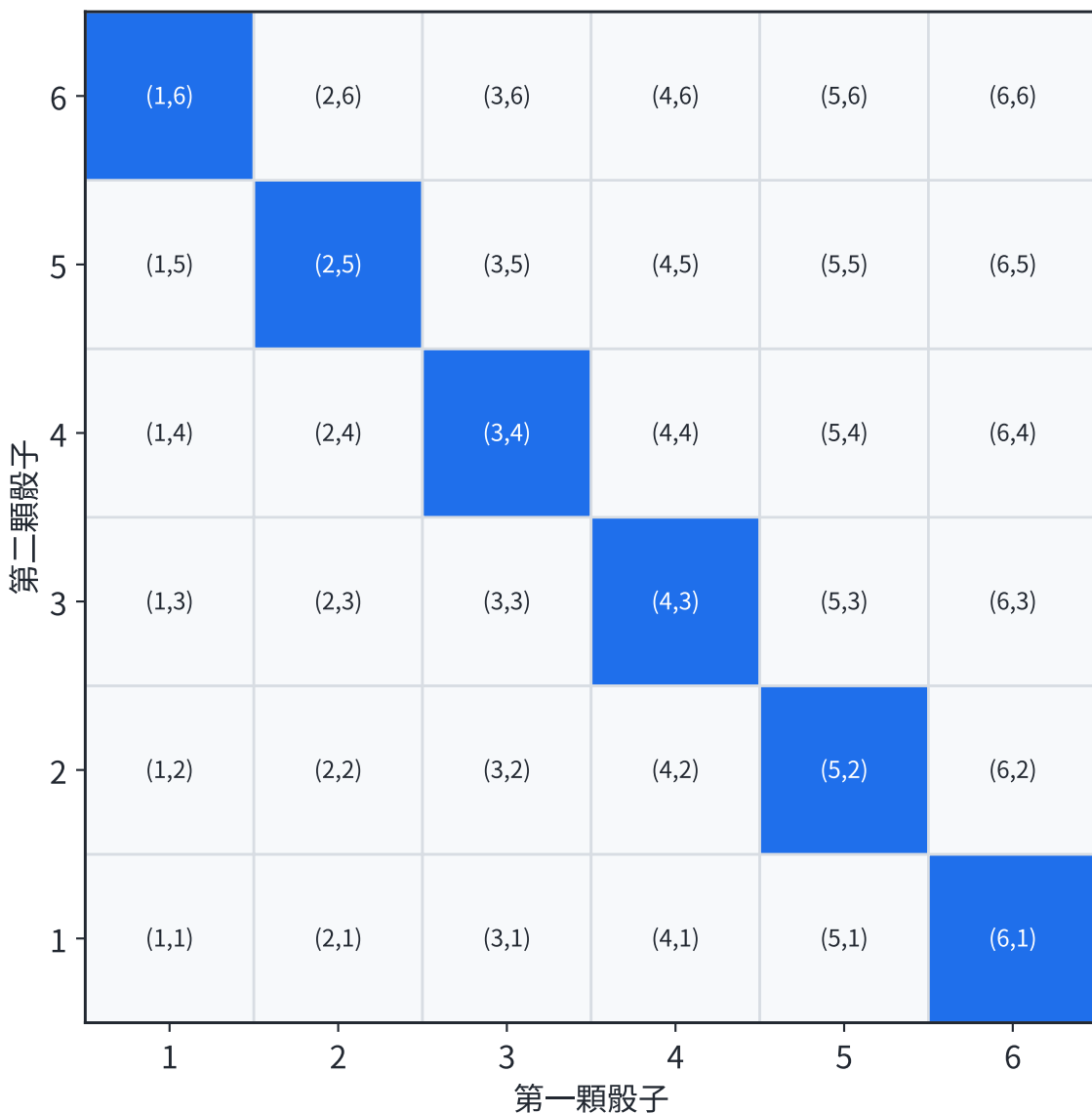
兩顆公平骰子的 36 個等可能樣本點；點數和 7 有 6 點
