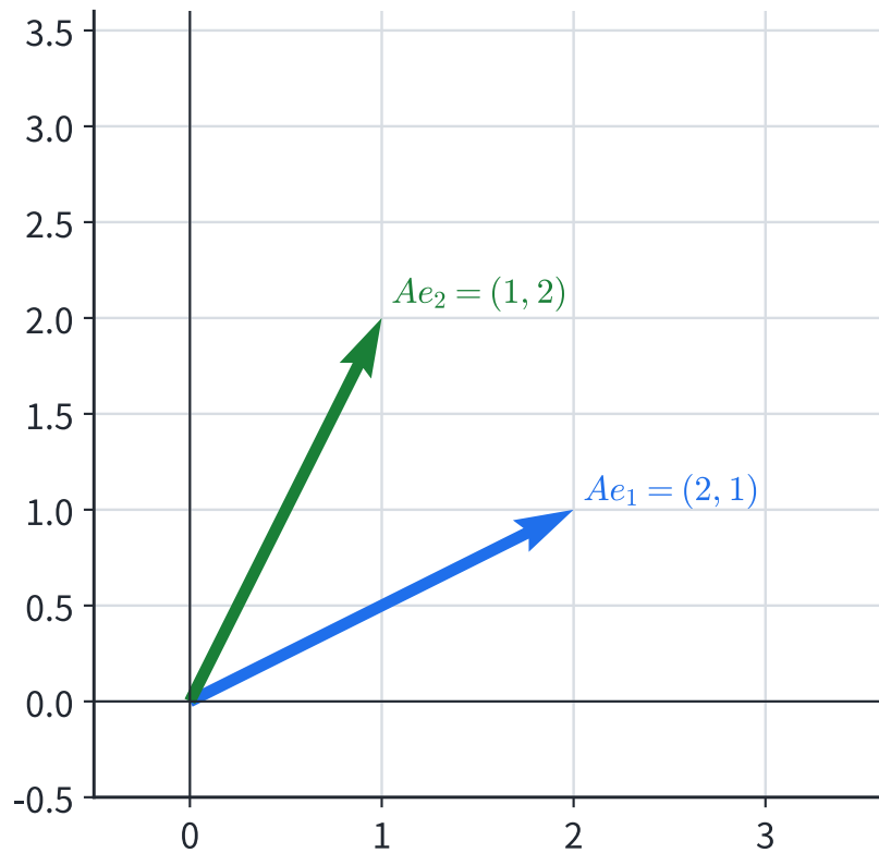
矩陣的兩個直行就是基底的像
