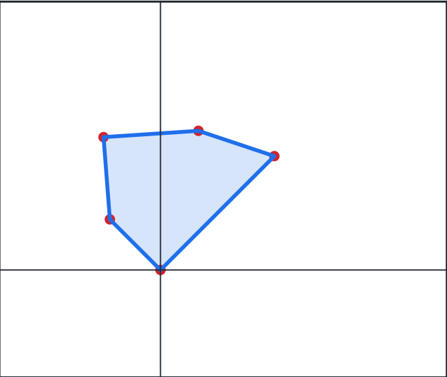
逆時針 45°
