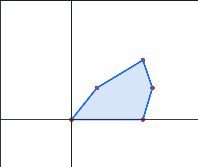
水平剪切
