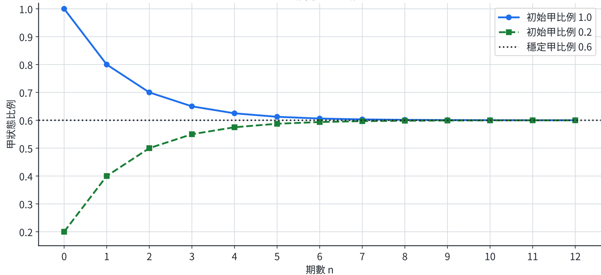
不同初始比例反覆使用 X_{n+1} = AX_n ，都接近同一穩定比例
