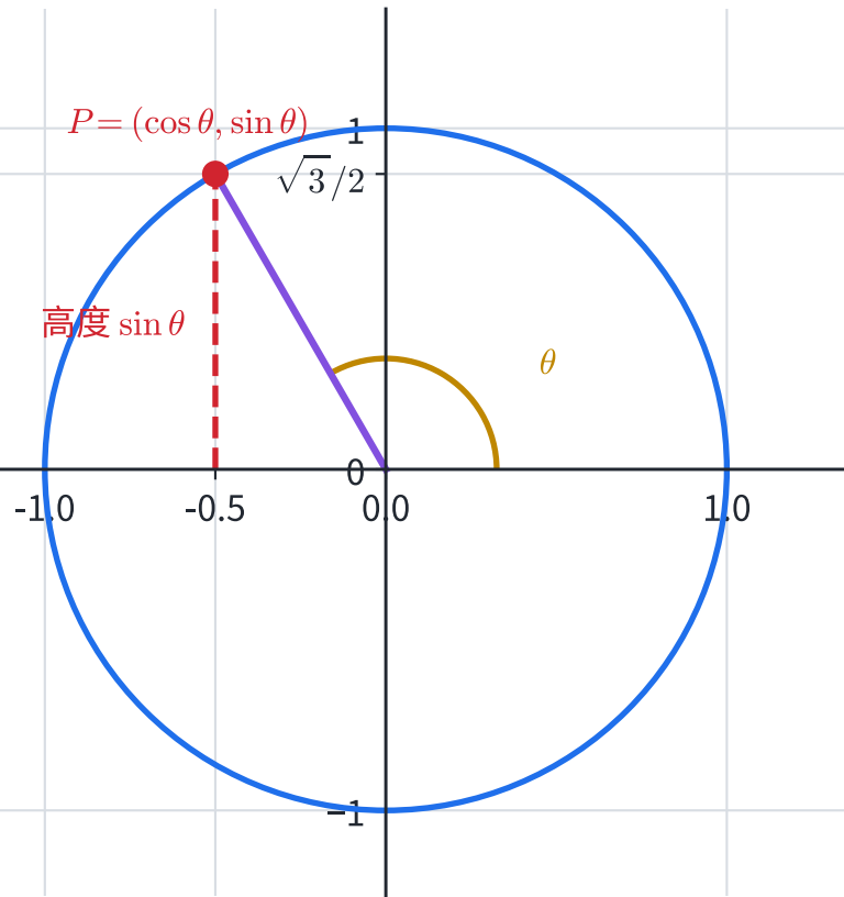
單位圓上的高度就是 \sin \theta
