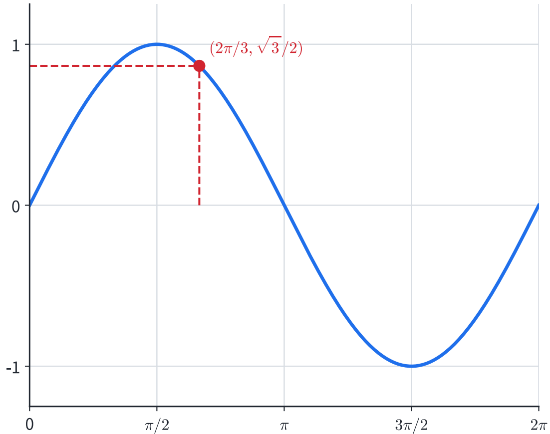
角度前進時，高度留下正弦圖形
