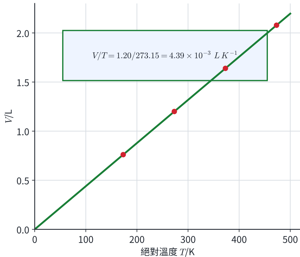
絕對溫度軸：比例直線過原點
