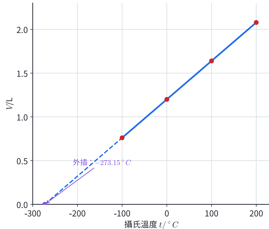
攝氏軸：直線外插到零體積
