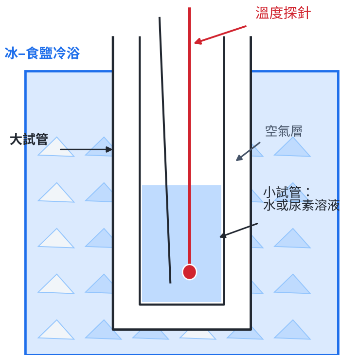
裝置控制熱傳與測溫位置
