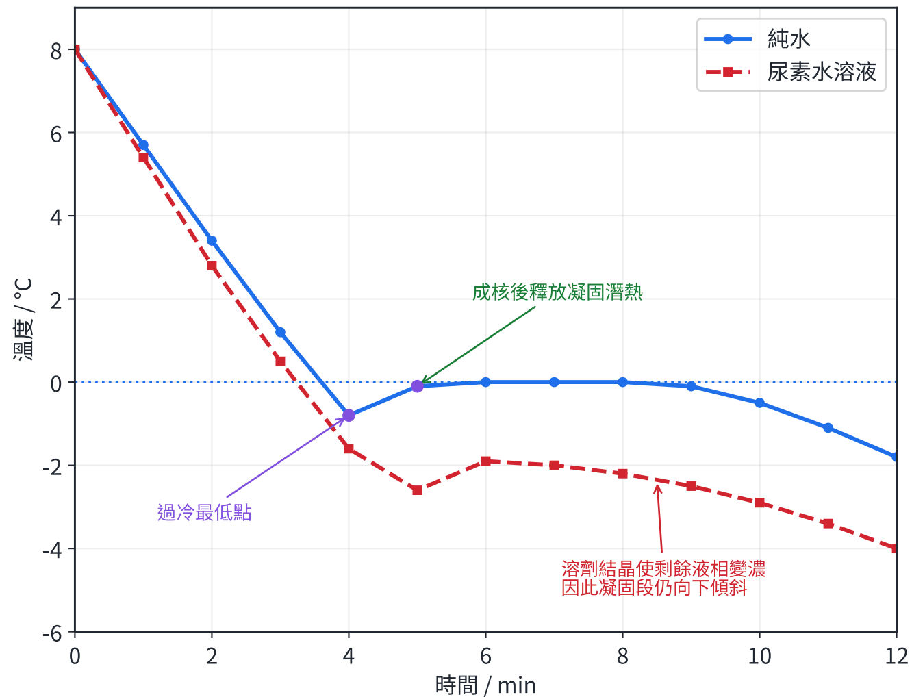
曲線形狀比單一最低點更能辨認凝固點
