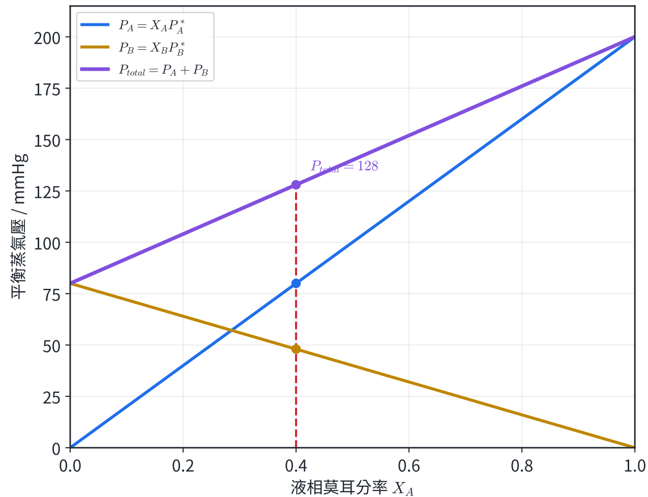
液相組成決定各成分分壓
