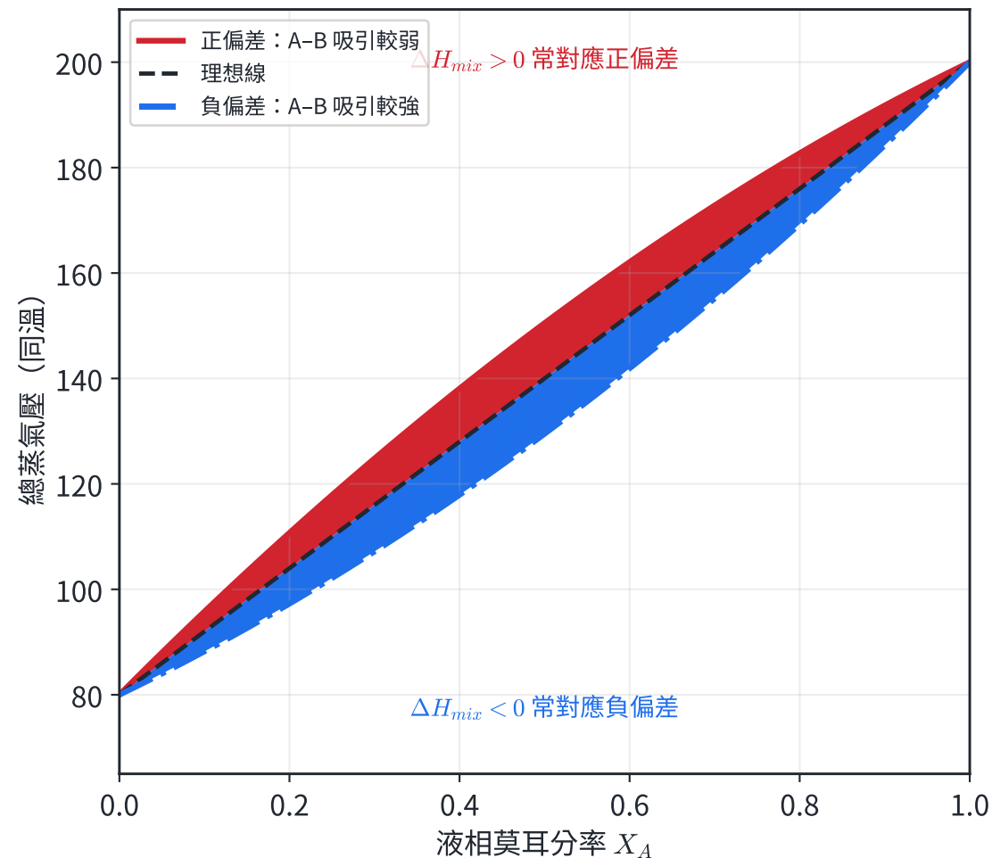
分子間作用力改變離開液面的難易
