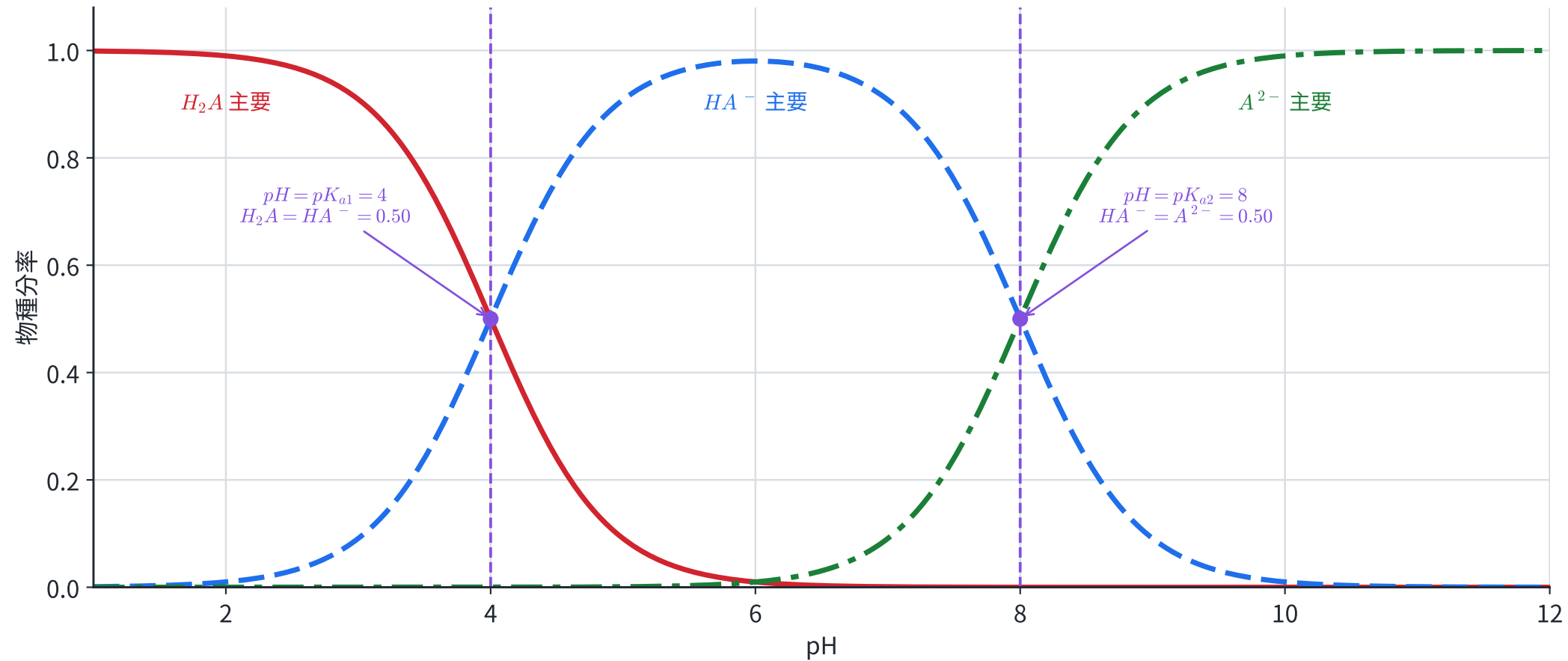
二質子酸 H_2A の物種分布 ( K_{a1} = 10^{-4} 、 K_{a2} = 10^{-8} )
