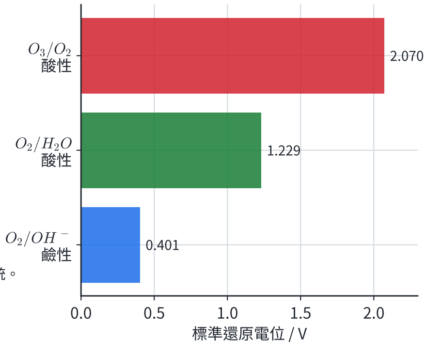
半反應條件改變氧化能力
