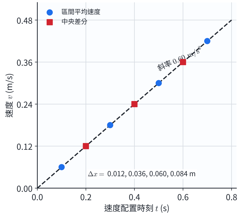
A | 第 15 題 兩種速度配置都給出相同斜率
