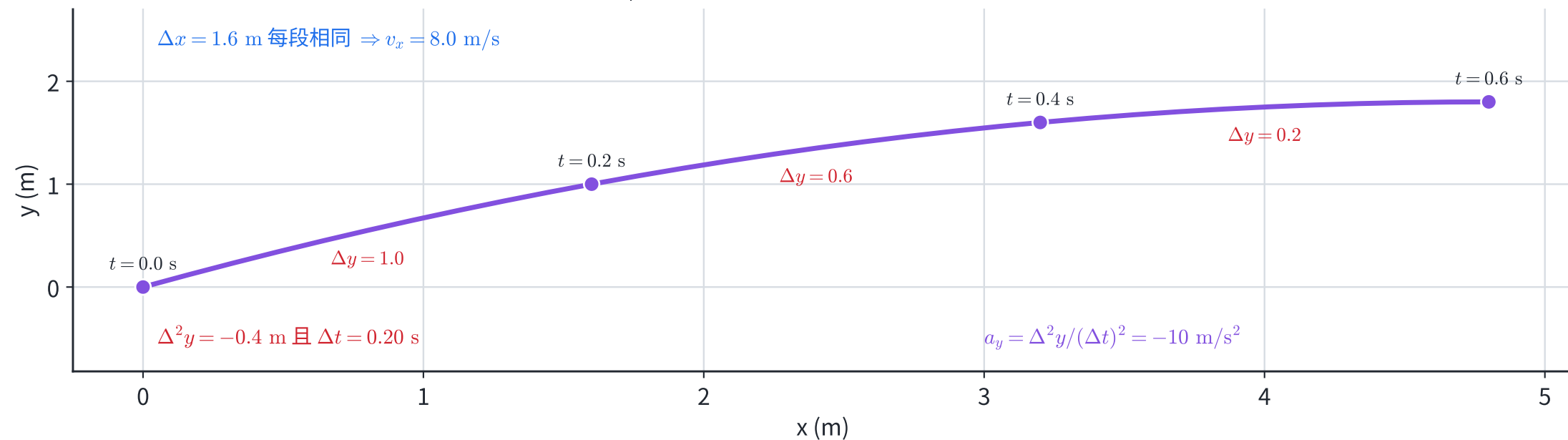
C | 第 15 題：等時距位置點重建加速度
