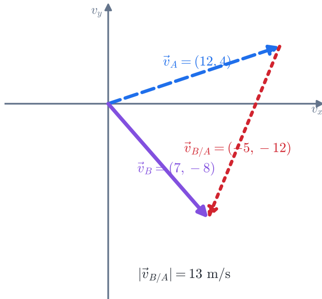
第 10 題 | \vec{v}_B = \vec{v}_A + \vec{v}_{B/A}
