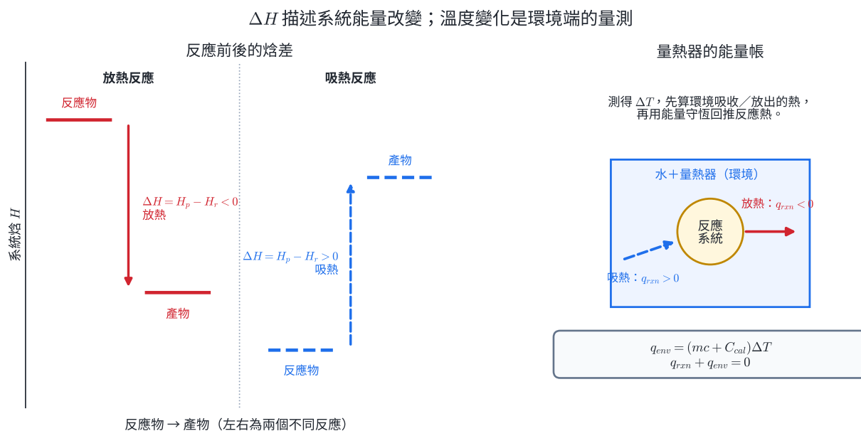
圖 7 | 左圖把放熱、吸熱分成兩個反應前後焓階；右圖以箭頭表示熱進出反應系統，量到環境溫度變化後由 q_{\text{rxn}} = -q_{\text{env}} 回推反應熱。
