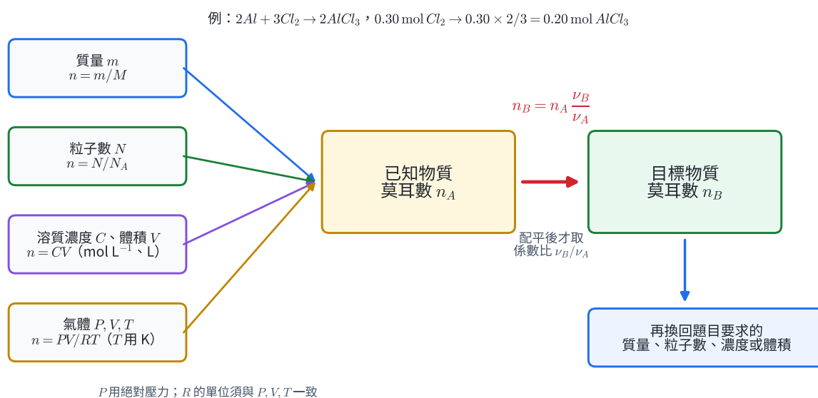
圖 4 | 質量、粒子數、溶液與氣體資料先換成莫耳數，再用配平係數比連到目標物；濃度與體積、氣體壓力與溫度須使用相容單位。
