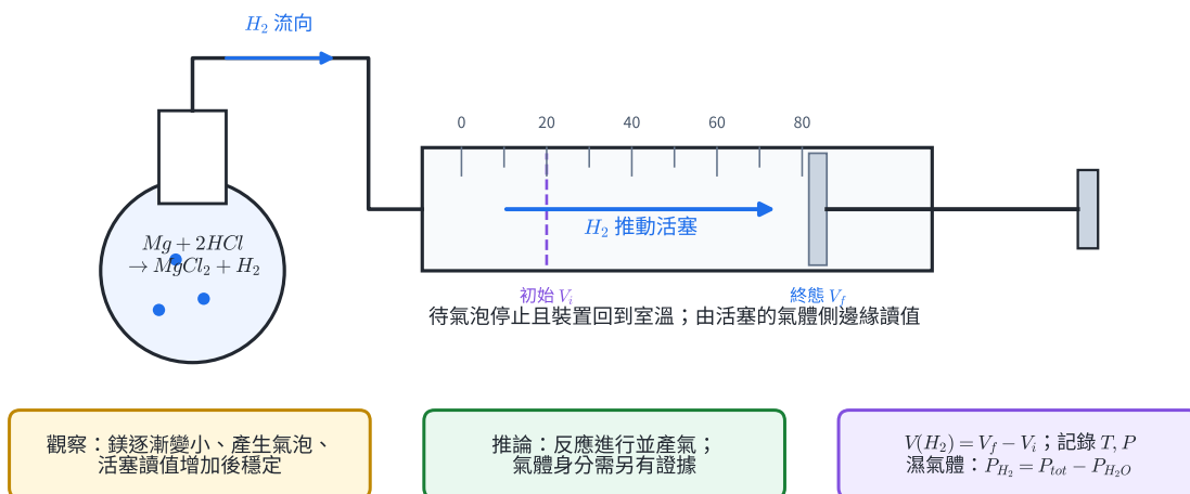
圖 6 | 氫氣由反應瓶流入氣體注射筒並推動活塞；回到室溫後由活塞的氣體側邊緣讀值，以 V_f - V_i 求產氣體積。
