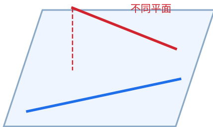
圖 1 | 空間位置關係。歪斜線的判斷同時用到「沒有交點」與「不共平面」。
