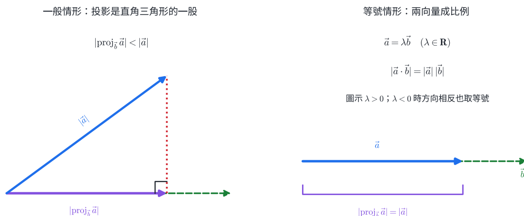
圖 7 | 一般情形的投影短於原向量；兩向量成比例時，投影長等於原向量長，柯西不等式取等號。
