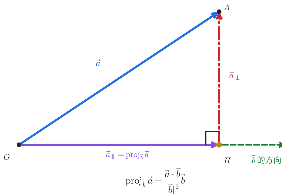
圖 6 | \vec{a} 分成平行於 \vec{b} 的投影與垂直於 \vec{b} 的剩餘分量。
