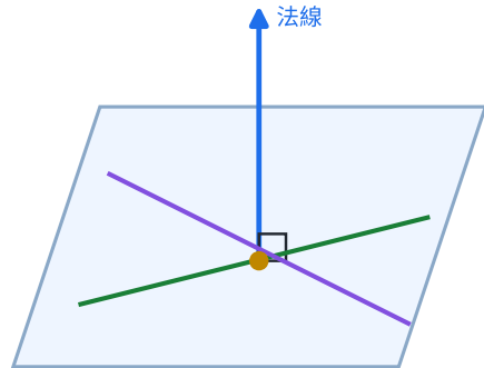
直線垂直平面
