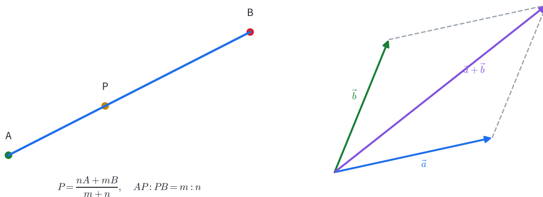
圖 4 | 左：內分點是端點的加權平均；右：向量加法逐分量進行。
