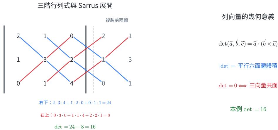
圖 9 | 三階行列式的計算與幾何意義。符號保留三個方向的排列順序。
