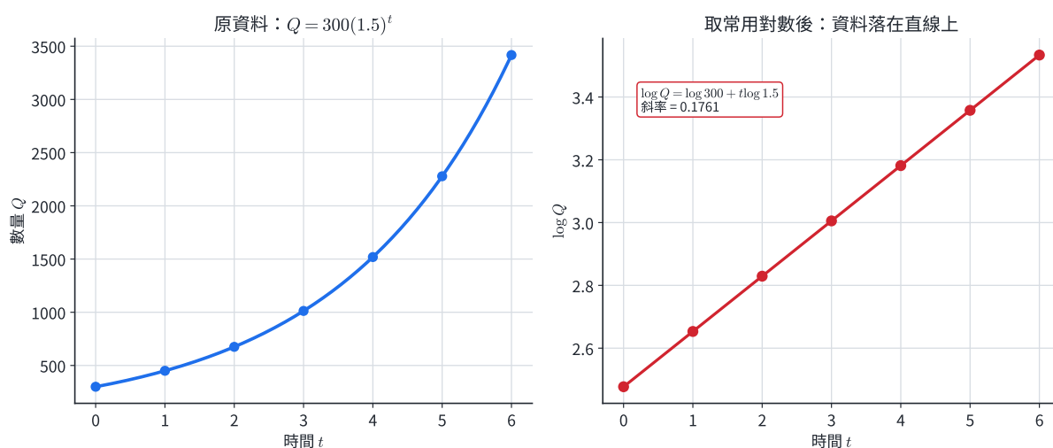
指數資料取常用對數後形成直線
