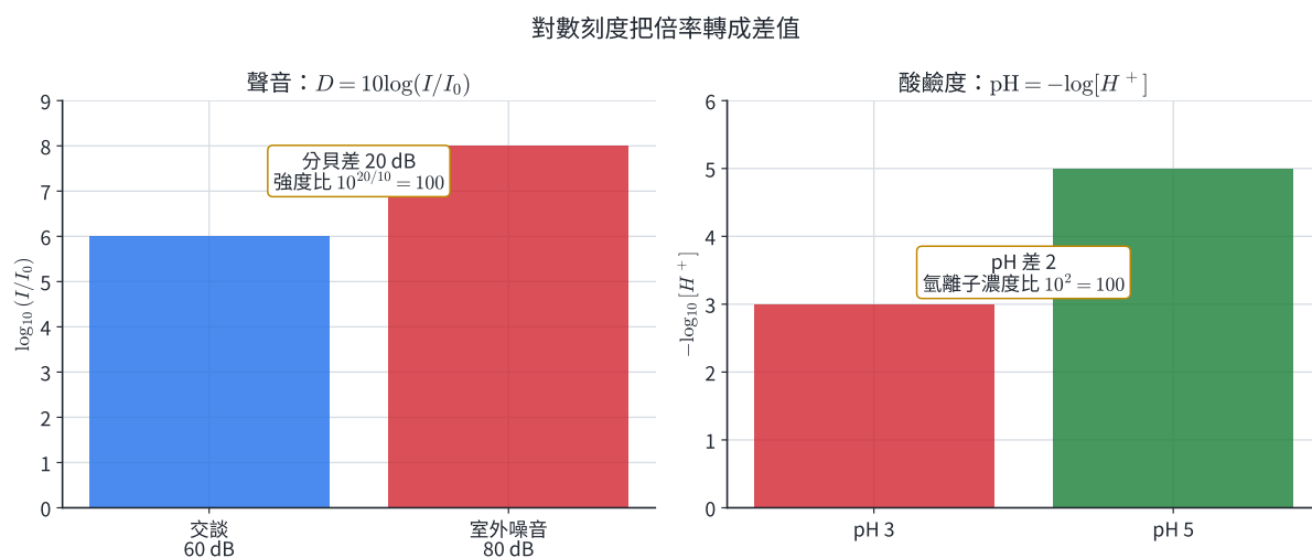
聲強與氫離子濃度在對數尺度上的對應
