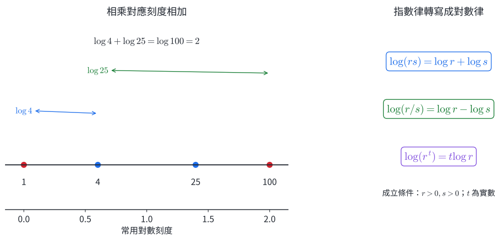
對數將乘法倍率轉成加法距離
