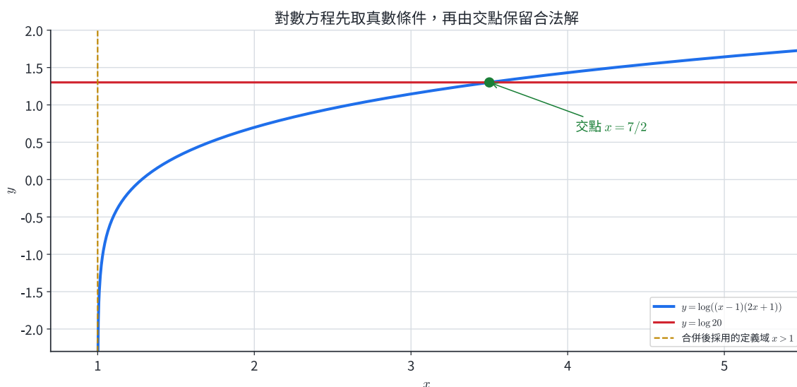
對數方程式的合法定義域與圖形交點
