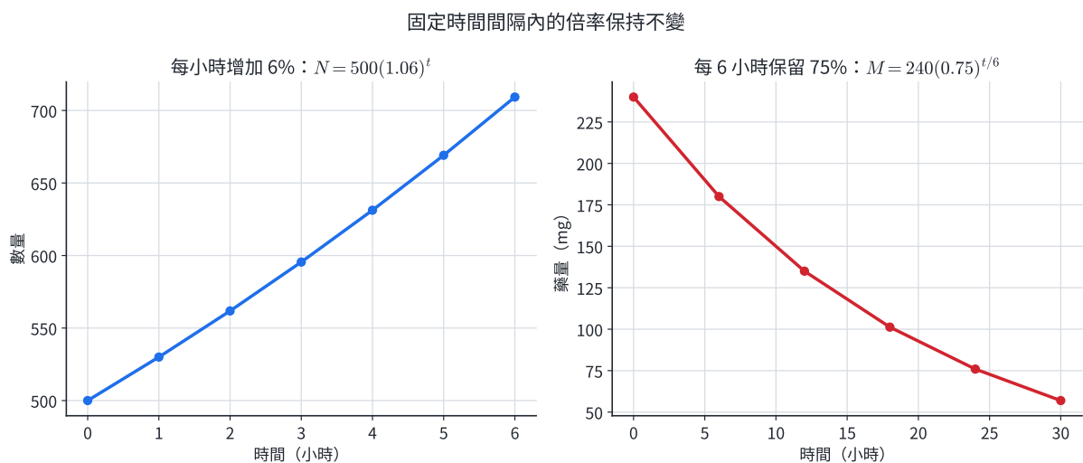
成長與衰退資料的固定時間倍率
