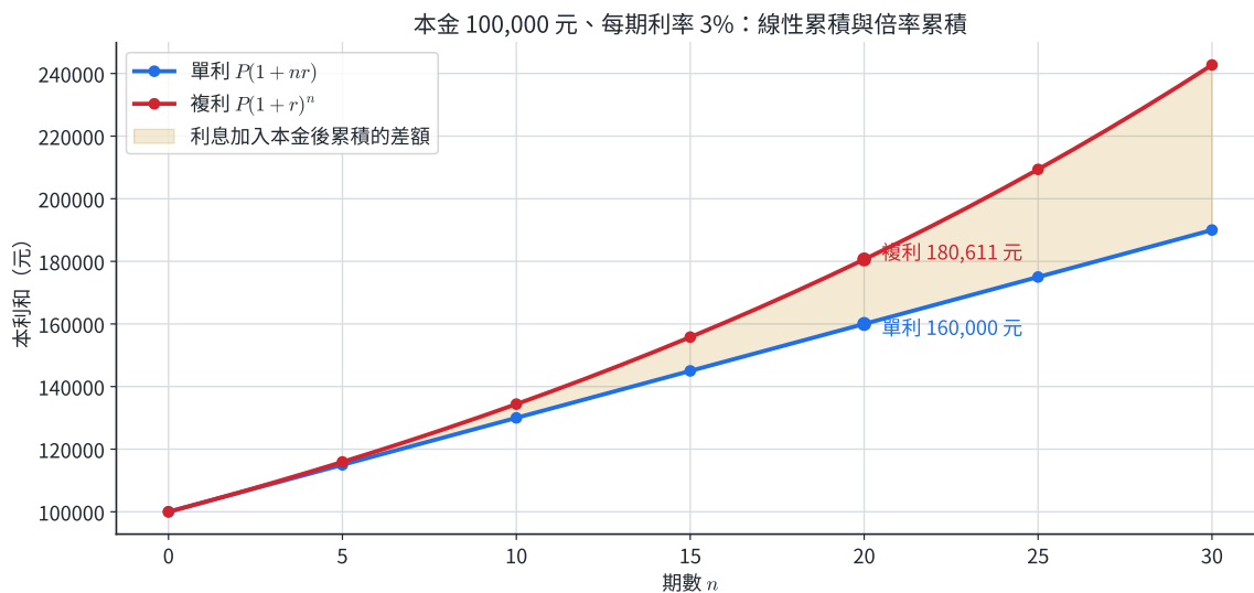
同一本金與利率下的單利、複利累積
