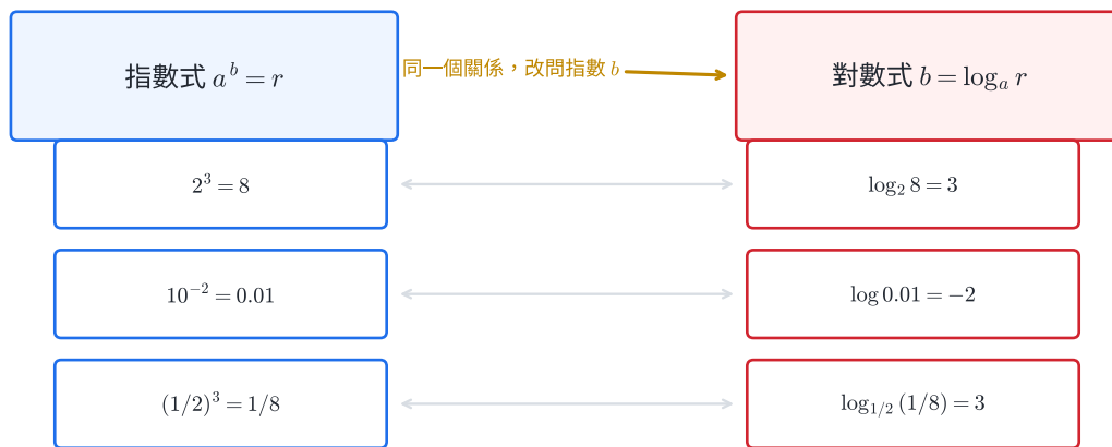
同一關係的指數形式與對數形式
