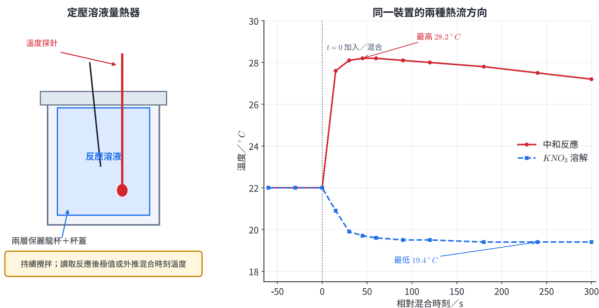
圖 6 | 保麗龍杯量熱器及兩組溫度—時間資料；兩組都以加入 / 混合時刻為 t = 0 ，中和曲線上升、硝酸鉀溶解曲線下降。
