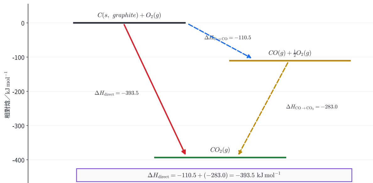
圖 5 | 碳完全燃燒的實線直接路徑與虛線兩步路徑具有相同初、終態； -110.5 + (-283.0) = -393.5 \text{ kJ mol}^{-1} 。
