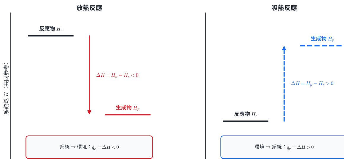
圖 4 | 放熱與吸熱反應使用同一焓參考；比較 H_p 與 H_r 的高低，垂直箭頭方向直接給出 \Delta H = H_p - H_r 的符號。
