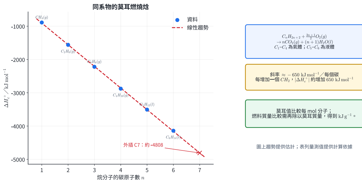
圖 8 | C_1 - C_6 直鏈烷在共同燃燒終態 CO_2(g) + H_2O(l) 下的標準莫耳燃燒焓；資料點標示反應物物態，虛線斜率估計每增加一個 CH_2 的影響。
