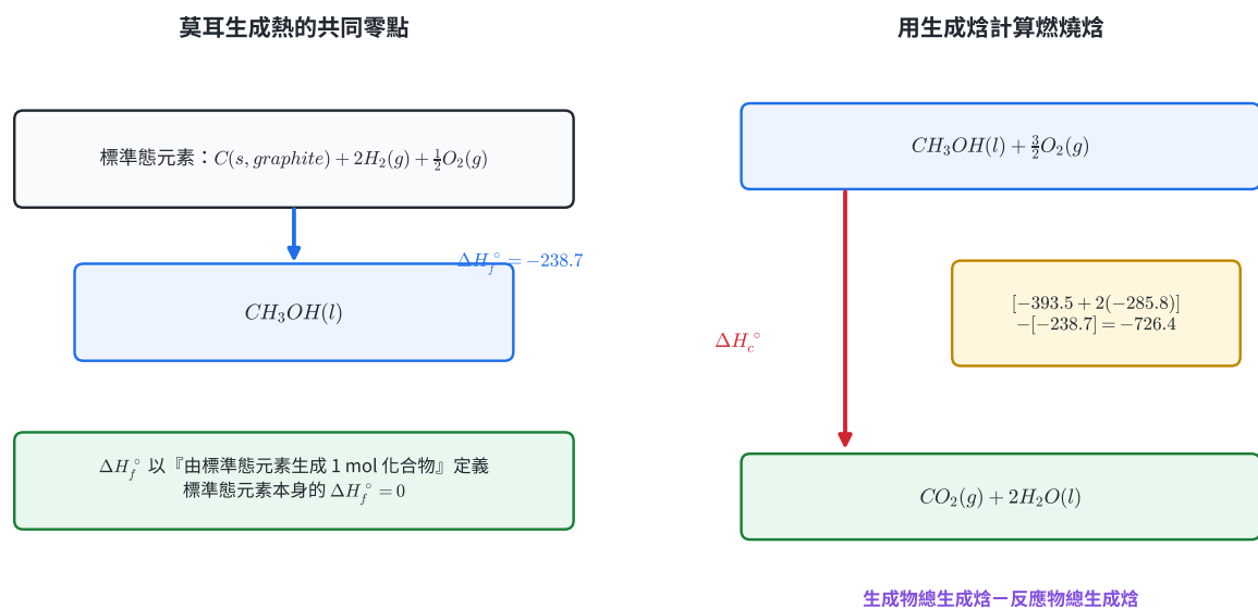
圖 7 | 標準態元素生成甲醇的路徑，以及甲醇完全燃燒到二氧化碳與液態水的共同能量帳。
