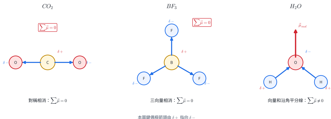
圖 8 | 藍箭頭是各鍵偶極，方向由 \delta+ 指向 \delta- ；紅箭頭是分子偶極向量和。CO 2 、BF 3 的對稱使總和為零，H 2 O 的兩個 H—O 鍵偶極都指向 O，向量和沿鍵角平分線。
