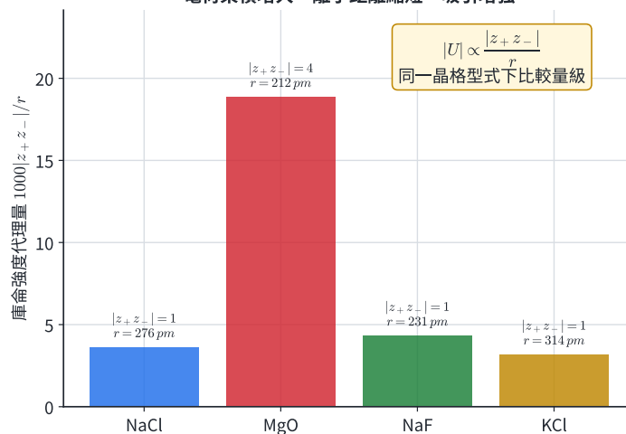
圖 2 | 左圖的正負離子數相等；右圖以電荷乘積除以距離比較四組離子的庫倫作用量級。
