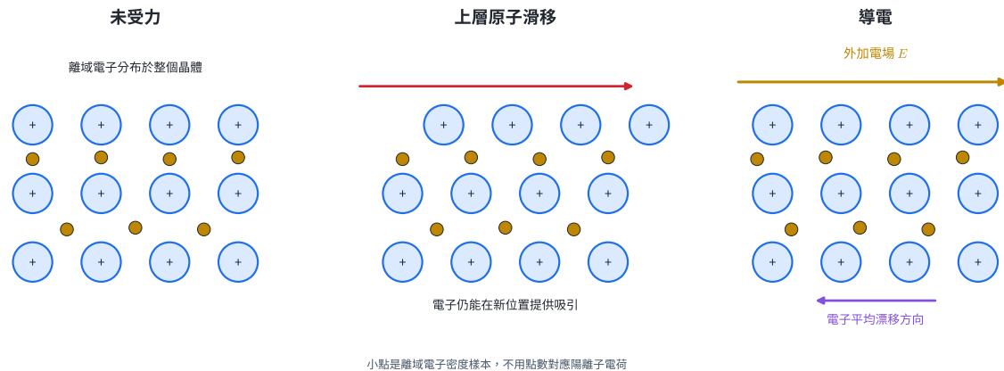
圖 3 | 晶格層滑移後，離域電子仍可提供吸引；外加電場時，電子平均漂移方向與電場方向相反。小點代表電子密度樣本。
