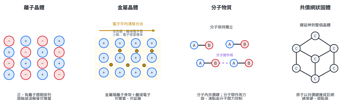
圖 4 | 先看粒子是離子、金屬陽離子、獨立分子或共價網，再由可移動電荷與連接範圍預測性質。金屬圖的小點是電子密度樣本；分子圖的虛線連接兩個實際分子。
