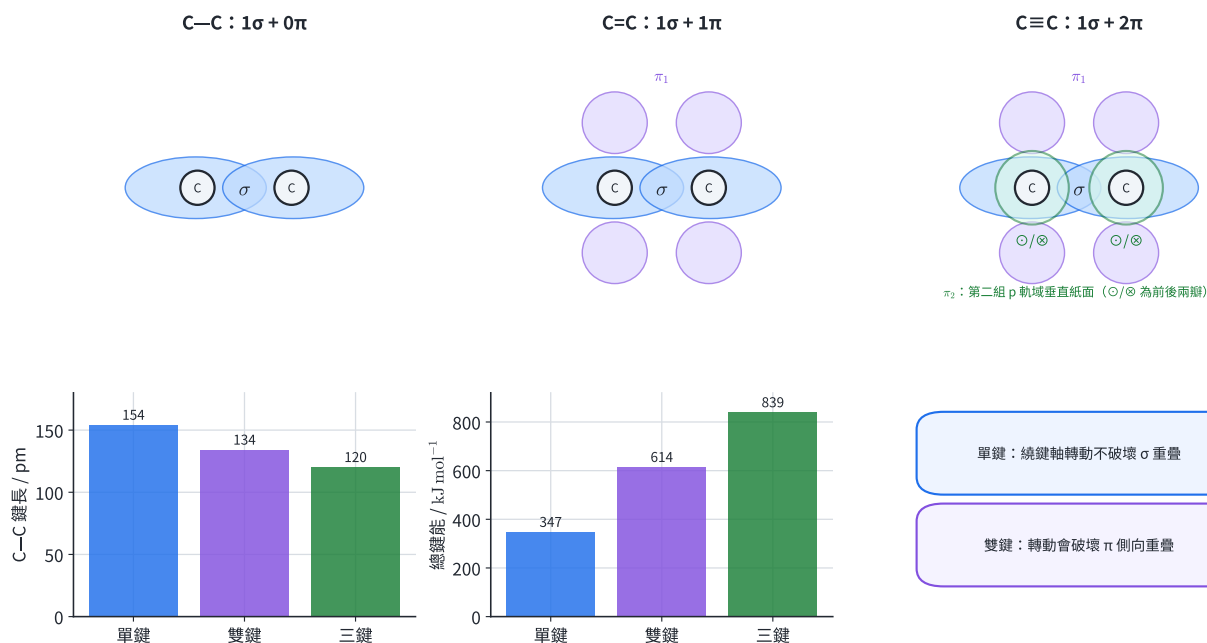
圖 5 | 上排由軌域重疊數出 \sigma 、 \pi ；三鍵中的 \odot/\otimes 表示每個 C 的第二組 p 軌域在紙面前後的兩瓣。下排標出同一組 C—C 鍵長與總鍵能數值。
