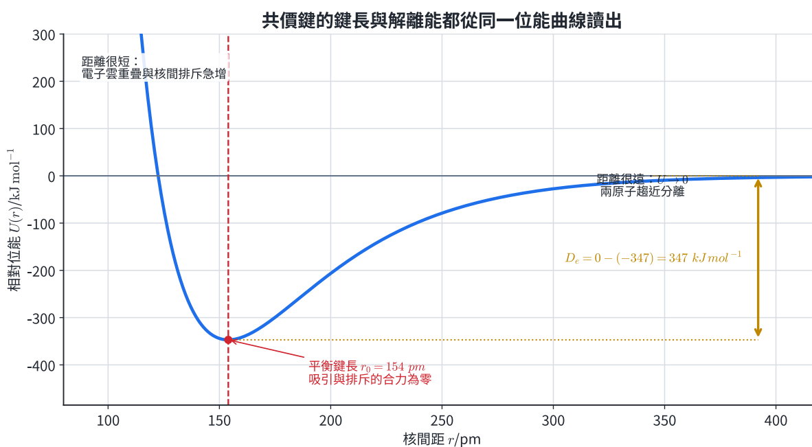
圖 1 | 沿曲線由右向左讀：原子由遠處靠近時位能先下降，在 r_0 最低；再壓近時排斥使位能急升。解離能是最低點到 U = 0 的垂直能量差。
