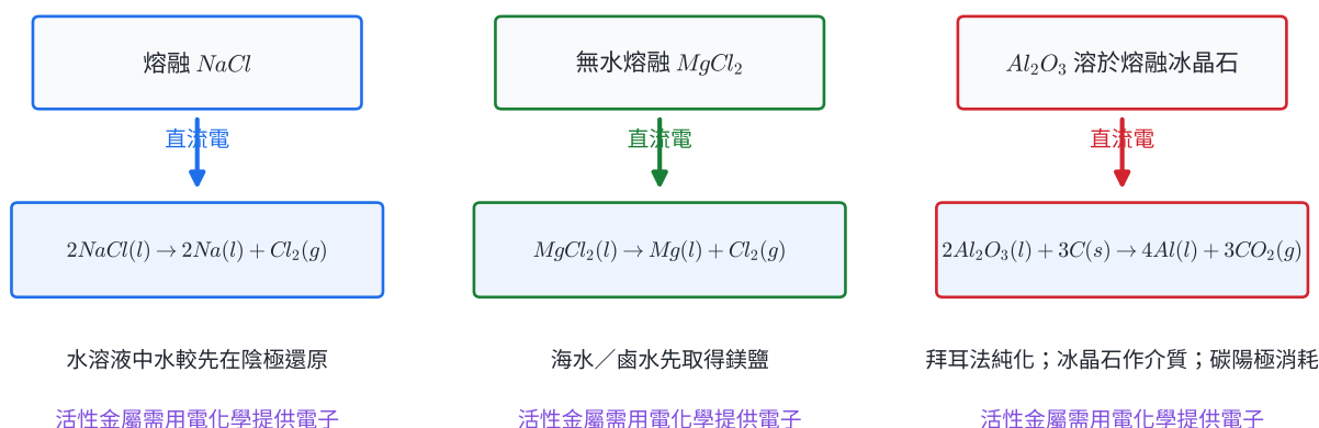
圖 6 | 鈉、鎂、鋁都由離子接受電子；原料純化與水的競爭決定熔融鹽製程。
