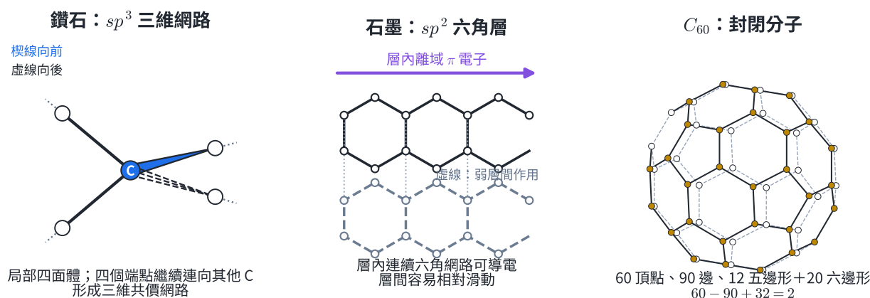
圖 2 | 鑽石的局部四面體連成三維網路，石墨烯六角網路堆疊成弱層間作用的石墨， \text{C}_{60} 則是 60 頂點的封閉分子。
