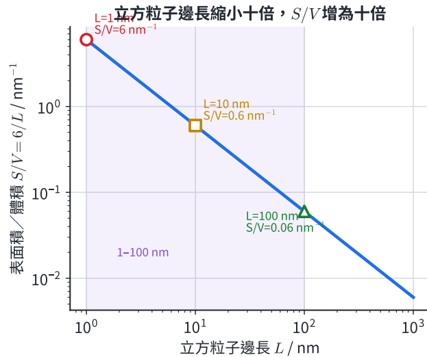
圖 13 | 左圖由 S/V = 6/L 計算尺寸效應；右圖由價帶到傳導帶的光激發，追蹤電子、電洞、表面反應與復合路徑。
