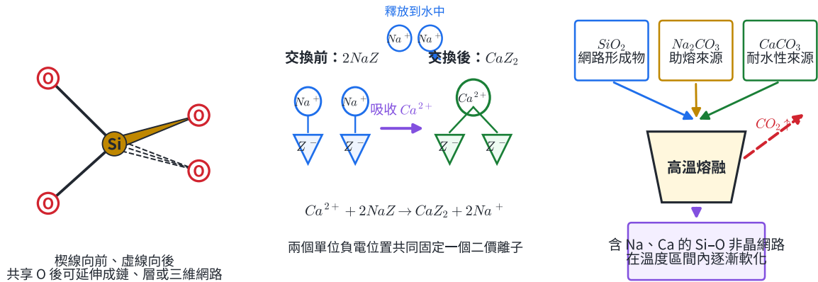
圖 5 | 矽氧四面體以楔線與虛線呈現立體鍵結；沸石以兩個單位負電位置交換一個 \text{Ca}^{2+} ，玻璃圖則追蹤入爐原料、Si-O 網路與 \text{CO}_2 流股。
