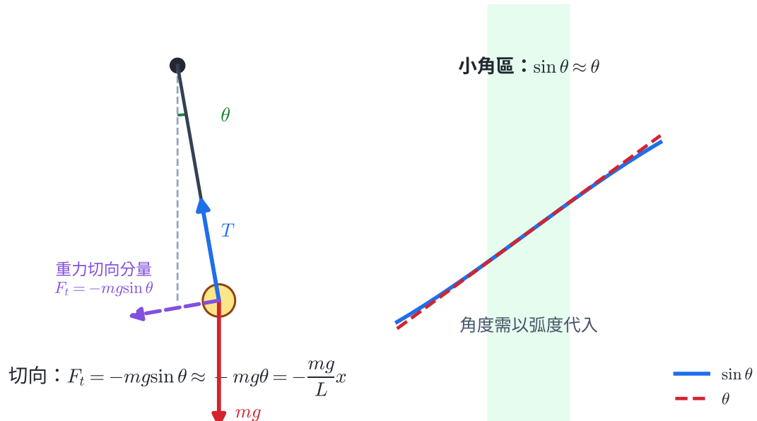
圖 7A | 紫色虛線是重力的切向分量 F_t = -mg \sin \theta ；圖中擺角 10^\circ 落在小角區。當 \theta 以弧度表示且角度小， \sin \theta \approx \theta = x/L 。
