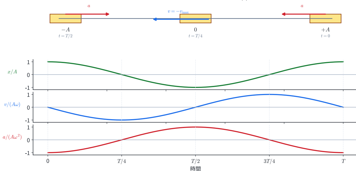
圖 6A | 取 t = 0 在 +A 靜止放開：第一次通過平衡點時 v = -v_{\max} ，到 -A 時速度再為 0。下圖以同一初始條件對齊 x 、 v 、 a 三條時間曲線。
