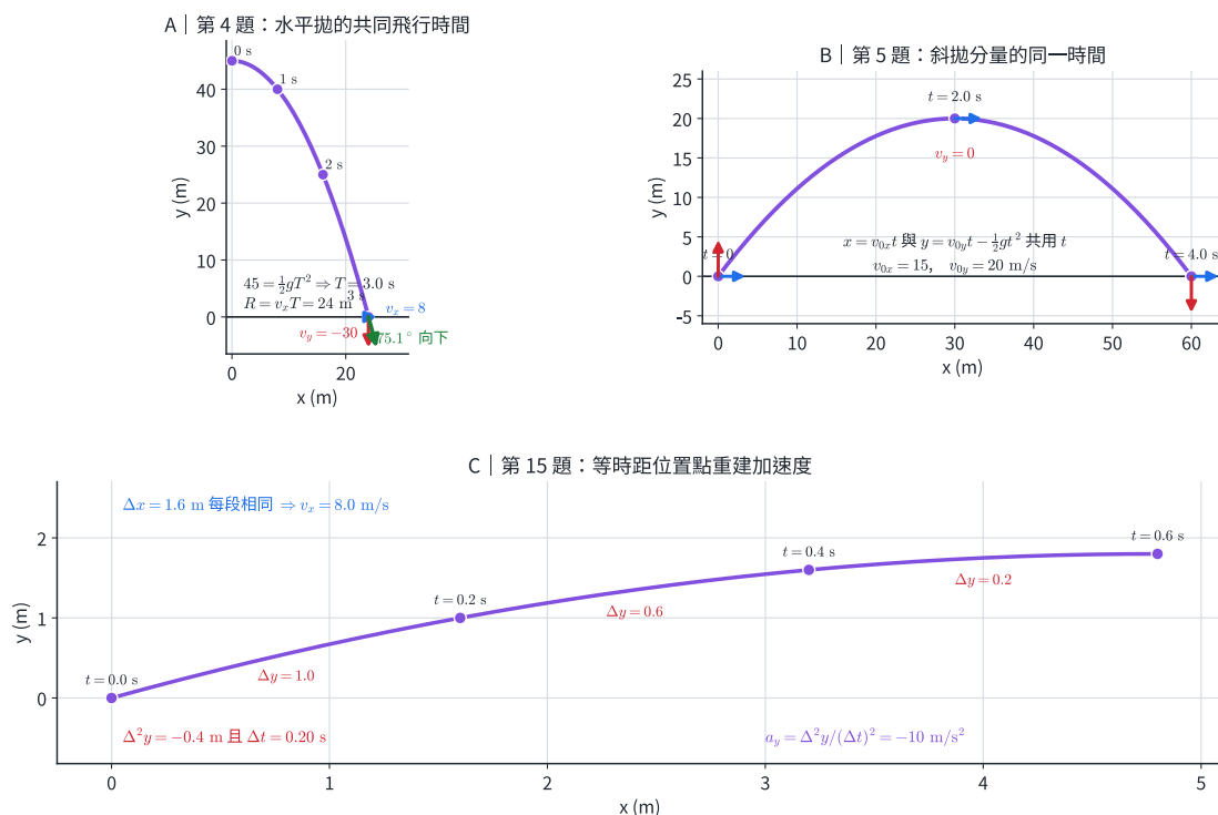
圖 7 | 章末第 4、5、15 題列式圖：A 用共同飛行時間連結水平拋的落下與水平位移；B 在同一時間下合成斜拋的水平、鉛直分量；C 從等時距位置點的一階與二階差分重建速度和加速度。
