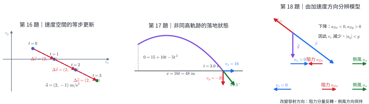
圖 11 | 章末第 16–18 題列式圖：A 在速度空間比較每秒的 \Delta \vec{v} ；B 以非同高軌跡的落地點求位移與速度方向；C 以加速度方向連結軌跡偏離，並用改變發射方向的試次分辨側風與阻力。
