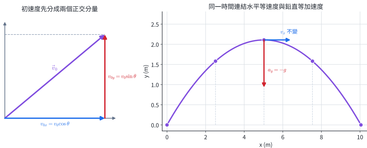
圖 4 | 拋體初速分成水平與鉛直分量；水平方向保持等速度，鉛直方向以 g 向下加速。
