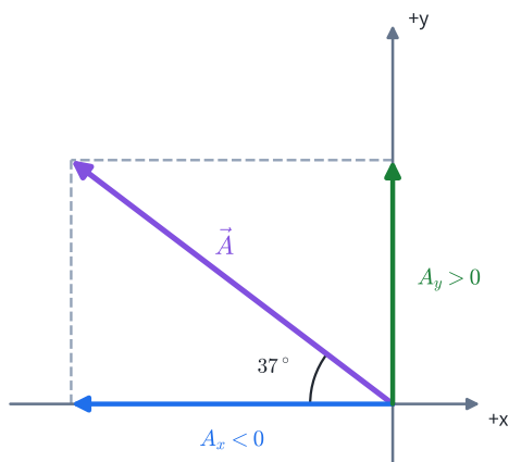
圖 1 | 先由箭頭方向判斷分量正負，再用直角三角形求量值；指向左上方時 A_x < 0 、 A_y > 0 。
