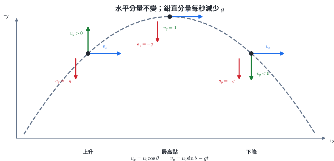
圖 5 | 理想拋體的水平速度分量全程不變；鉛直速度分量在上升時為正、最高點為零、下降時為負，而鉛直加速度全程為 -g 。
