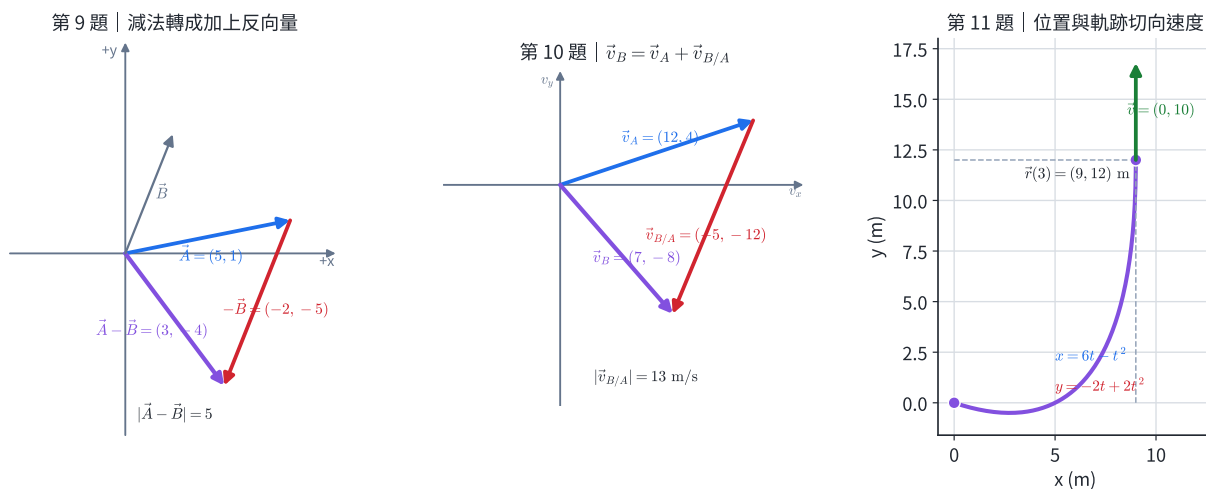
圖 9 | 章末第 9-11 題列式圖：A 將減向量轉成加上 -\vec{B} ；B 以 \vec{v}_B = \vec{v}_A + \vec{v}_{B/A} 建立相對速度；C 從位置軌跡的終點與切向讀出 \vec{r}(3) 與 \vec{v}(3) 。
