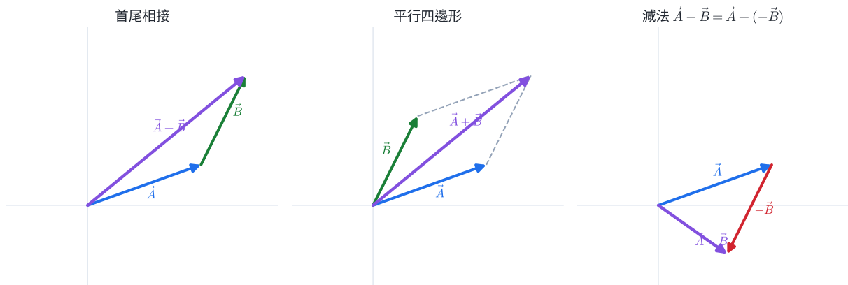
圖 2 | 首尾相接與平行四邊形得到同一個 \vec{A} + \vec{B} ；相減先把 \vec{B} 反向，再作 \vec{A} + (-\vec{B}) 。
