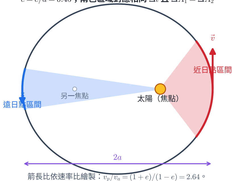
圖 4A | 橢圓軌道的太陽位於一個焦點；紅、藍區域對應相同時間，面積相等，而近日點軌道弧較長。
