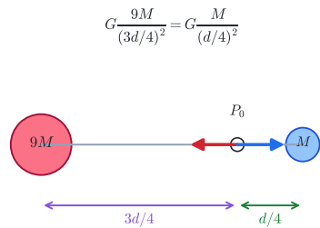
G | Q11：零場點的方向與距離
