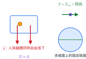
E | Q8：受力與軌道幾何
