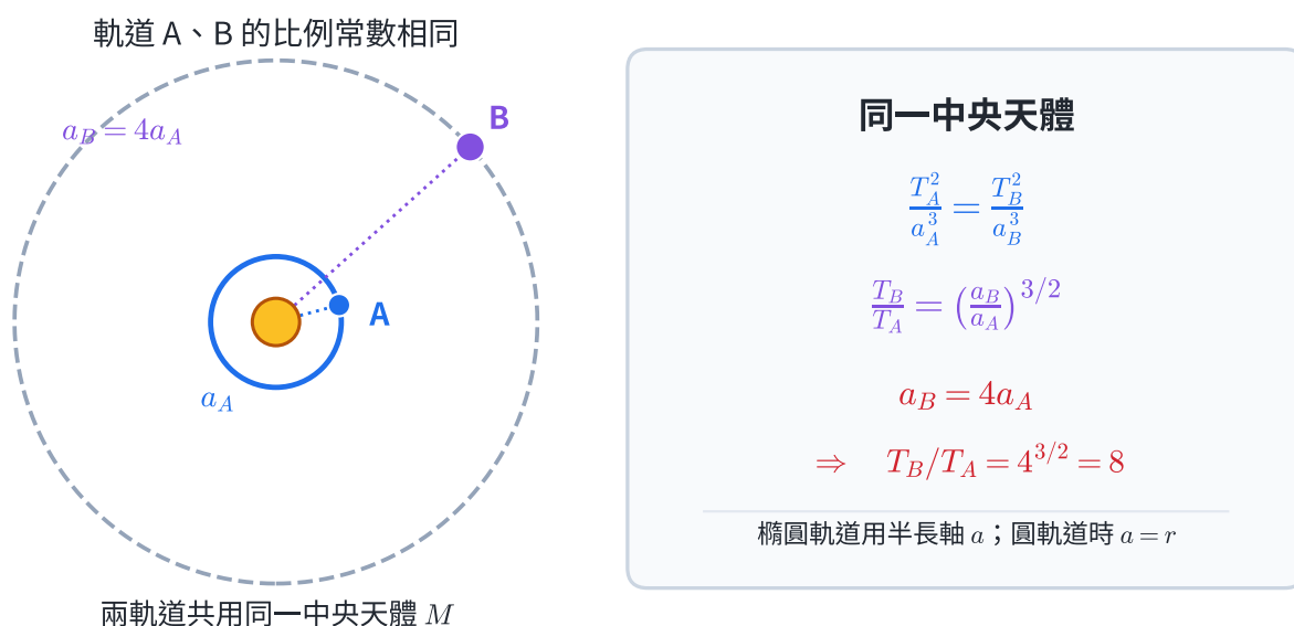
圖 4 | 同繞中央天體 M 時，軌道 B 的半長軸若為 A 的 4 倍，週期就是 8 倍；圓軌道以 r 代替 a 。
