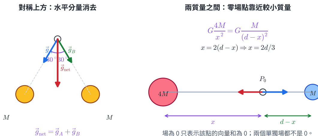
圖 3A | 左圖的兩個等質量場在對稱點水平分量消去；右圖的零場點位於 4M 與 M 之間，且靠近較小質量。
