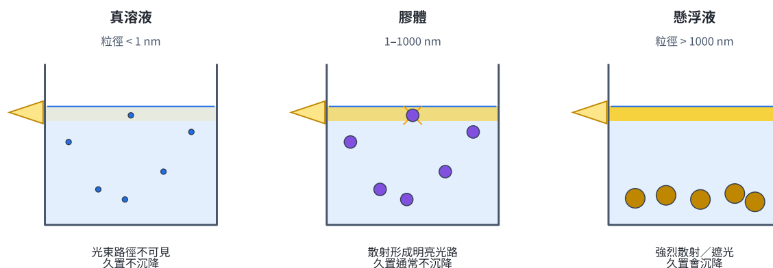
圖 1 | 真溶液、膠體與懸浮液的粒徑改變散射與沉降行為；光路是否可見是粒徑證據。
