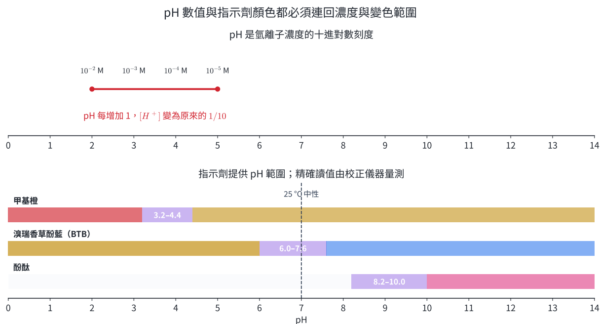
圖 6 | pH 每改變 1 對應氫離子濃度的十倍差；指示劑的呈色只限制 pH 落在某一範圍。
