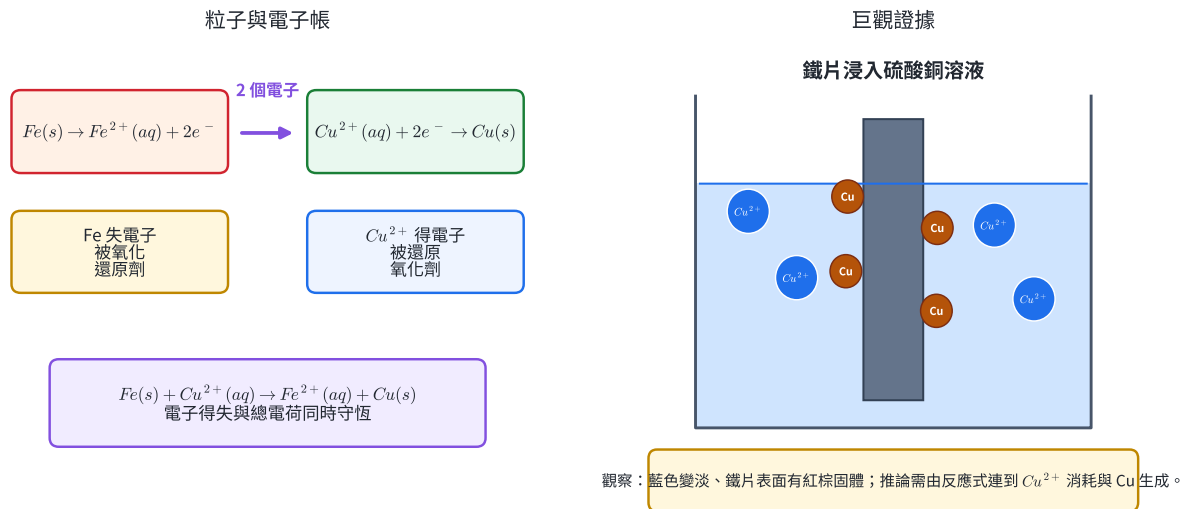
圖 8 | 鐵失去兩個電子、銅離子得到兩個電子；電子帳連到藍色變淡與銅析出的巨觀證據。
