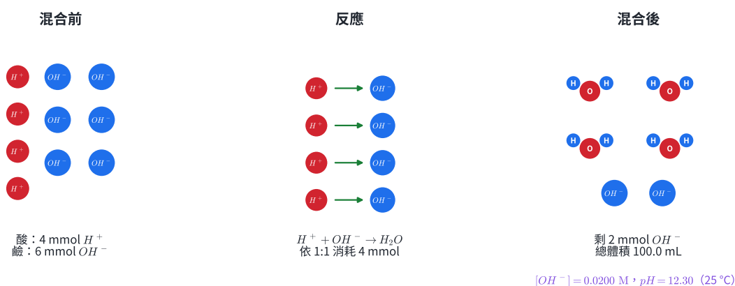
圖 7 | 4.0 mmol H^+ 與 6.0 mmol OH^- 反應後剩 2.0 mmol OH^- ；pH 由剩餘量決定。
