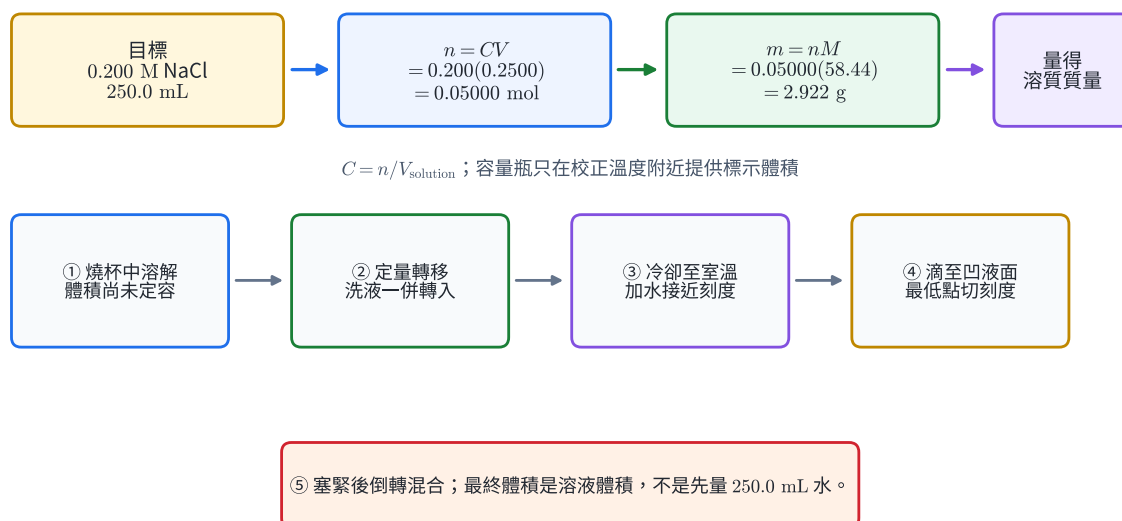
圖 2 | 配製 0.200 M NaCl 250.0 mL 的數量計算與定量轉移流程。
