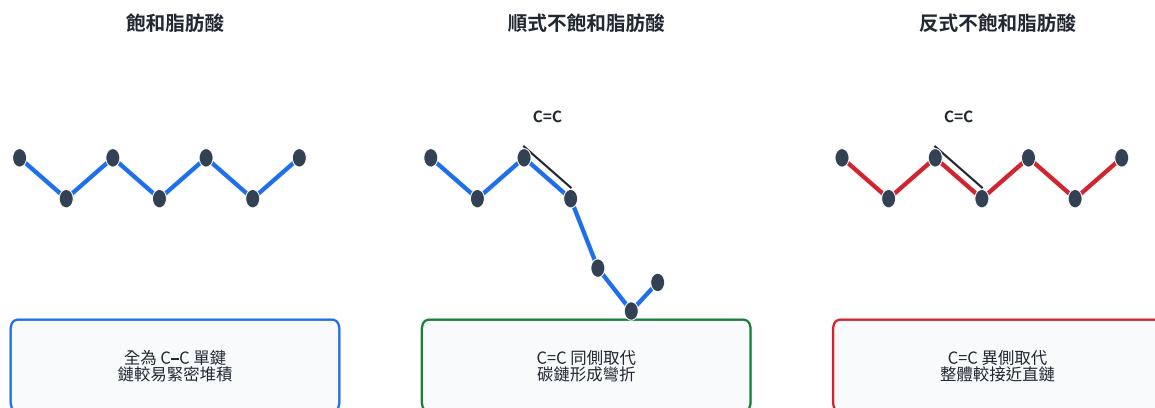
圖 2 | 飽和、順式與反式脂肪酸的鍵型和幾何；鍵形改變堆積效率。
