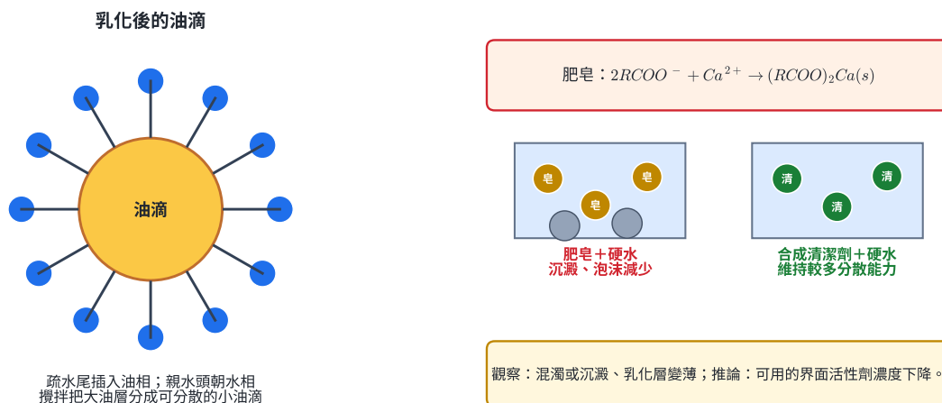
圖 3 | 微胞方向與硬水實驗的證據鏈；沉澱使可用肥皂濃度下降。
