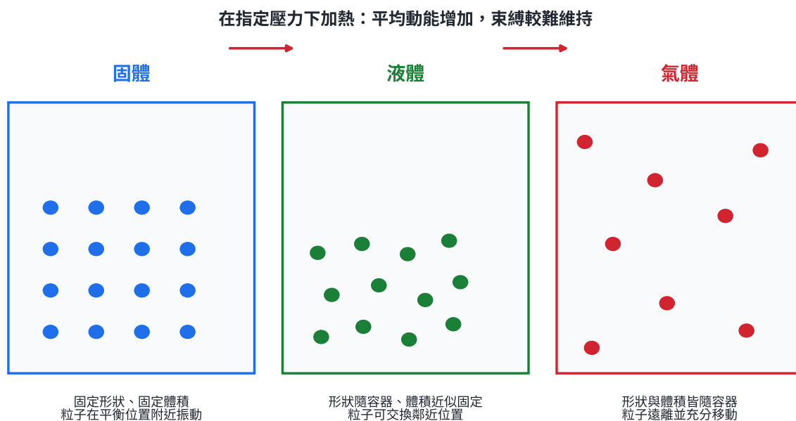
物質三態的粒子模型
