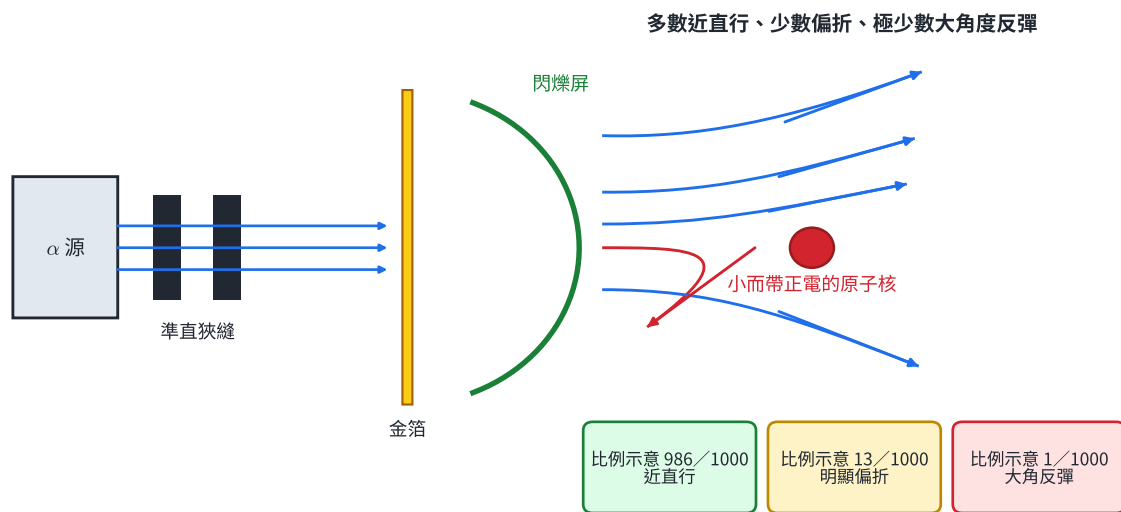
拉塞福散射與原子核
