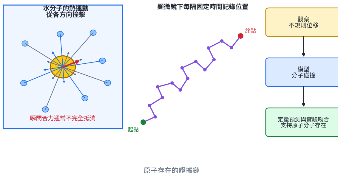
原子存在的證據鏈
