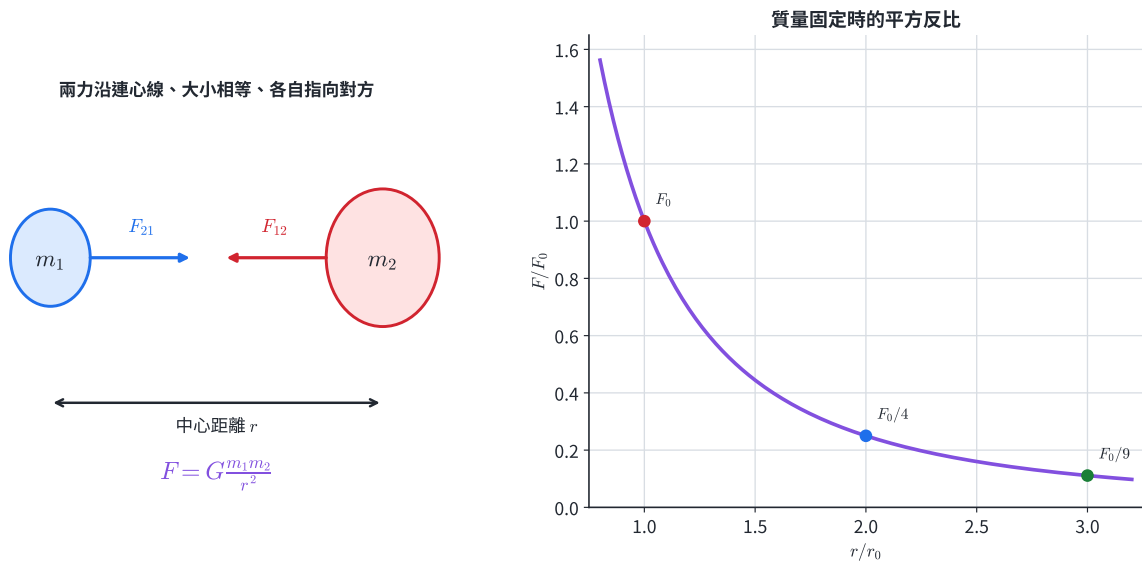
萬有引力與平方反比
