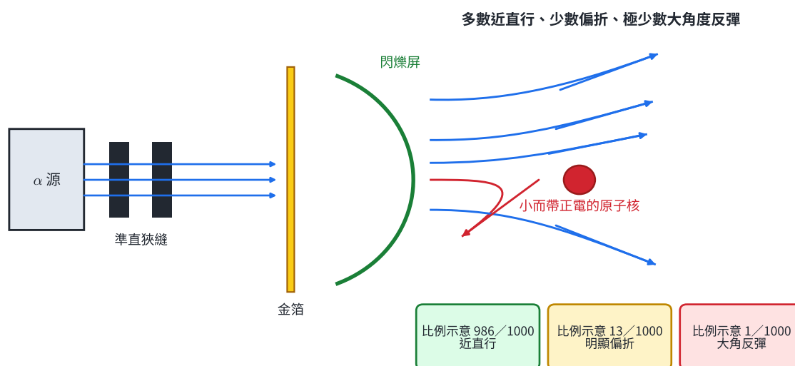
拉塞福散射與原子核
