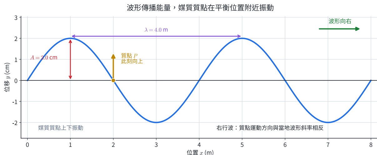
圖 8 | 振幅、波長、週期與質點運動方向；右行波在負斜率處的質點向上。
