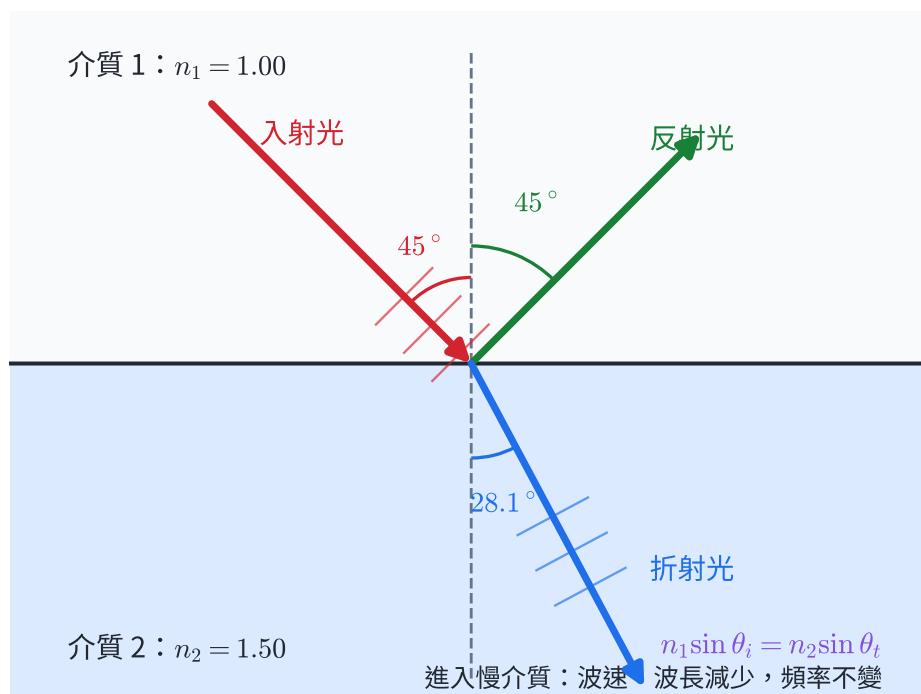
圖 9 | 反射角等於入射角；光由空氣進入折射率 1.5 的玻璃，入射角 45° 對應折射角約 28.1°。
