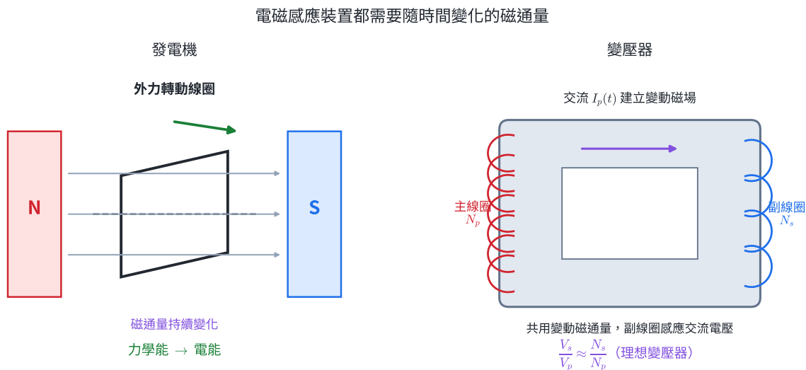
圖 4 | 發電機以轉動改變磁通量；變壓器以交變磁通量把能量耦合到次級線圈。
