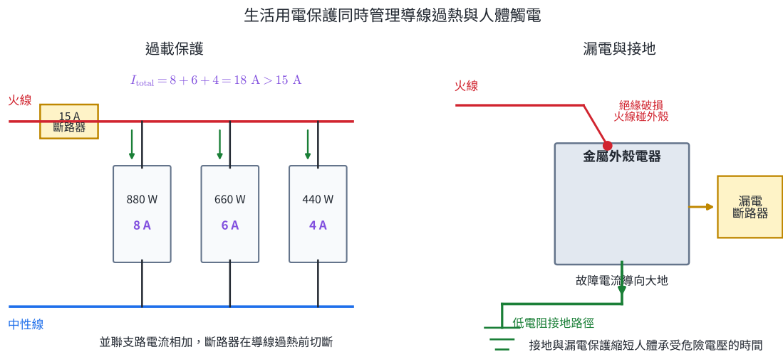
圖 5 | 家用支路並聯；過電流保護裝在火線，金屬外殼接地，漏電斷路器比較去回電流。
