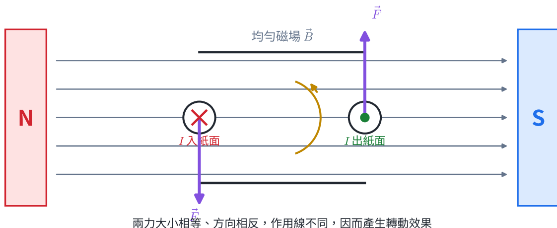
圖 2 | 磁場由 N 指向 S；左側電流入紙面而受力向下，右側電流出紙面而受力向上。
