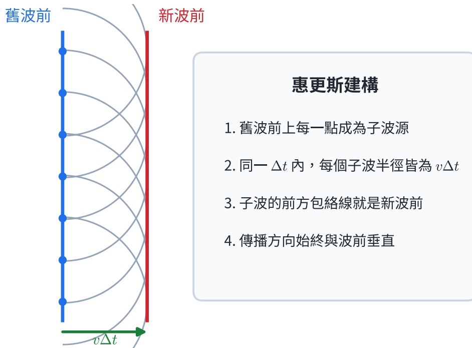
圖 10 | 波前上每一點都產生次波；下一時刻所有次波的包絡面形成新波前。
