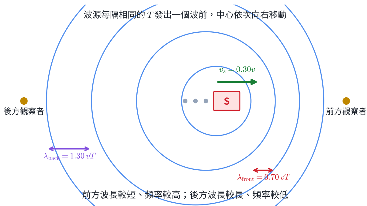
圖 12 | 波源向右移動，使前方波長縮短、接收頻率升高；後方波長拉長、接收頻率降低。
