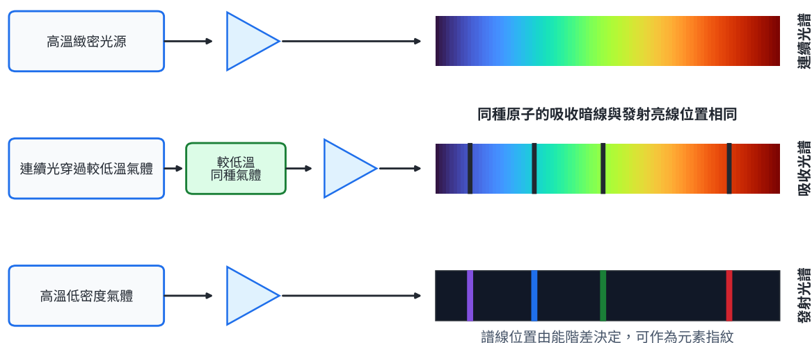
連續、吸收與發射光譜的形成路徑
