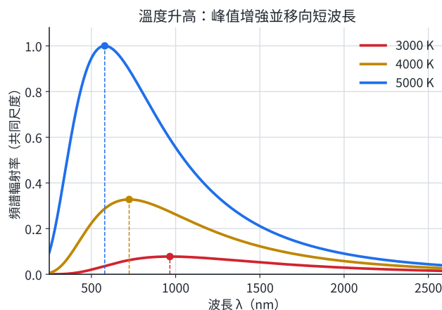
黑體輻射與能量量子化
