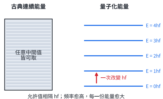
普朗克以離散能量交換描述輻射
