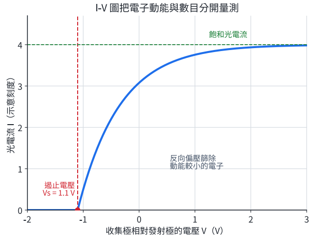
光電效應裝置與電流電壓
