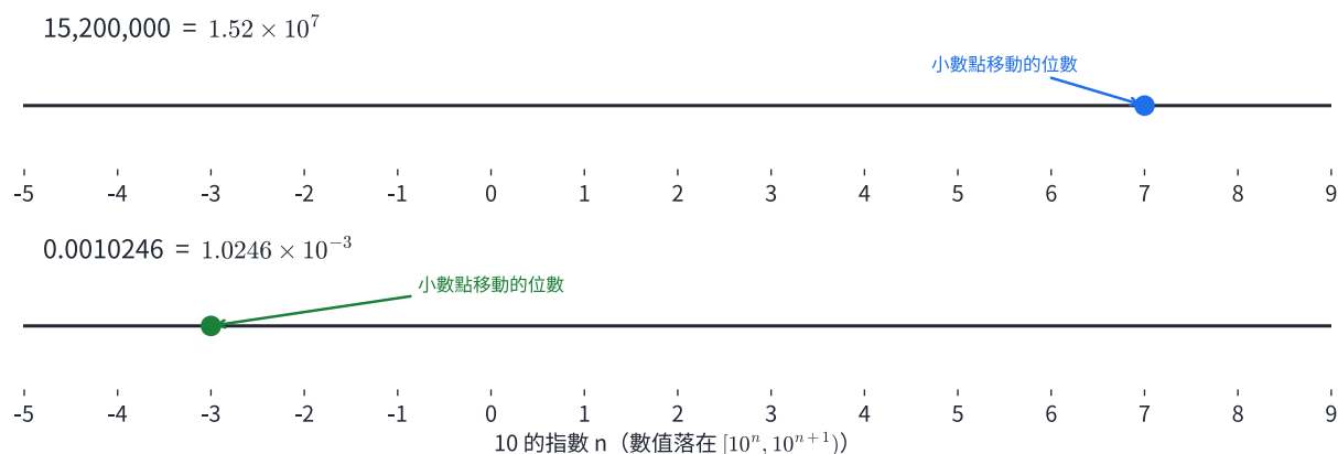
圖 3 | 科學記號的係數落在 1 到 10，指數標示原數所處的 10 倍區間。
