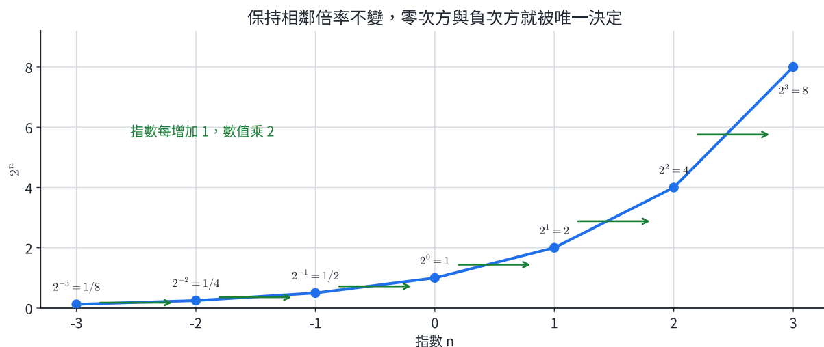
圖 1 | 相鄰指數相差 1 時，數值維持固定倍率；圖中的點由方程直接計算。
