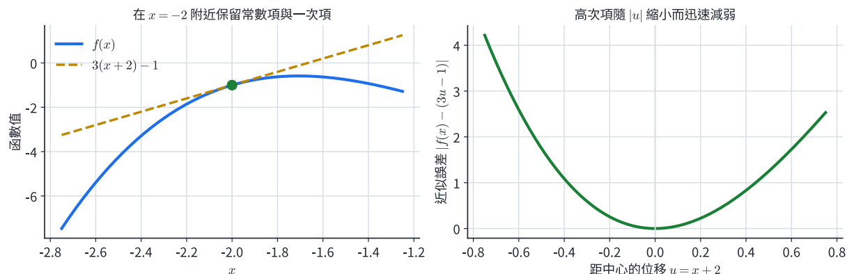
圖 10 | 左圖比較函數與一次近似，右圖直接畫出誤差隨位移增加的變化。
