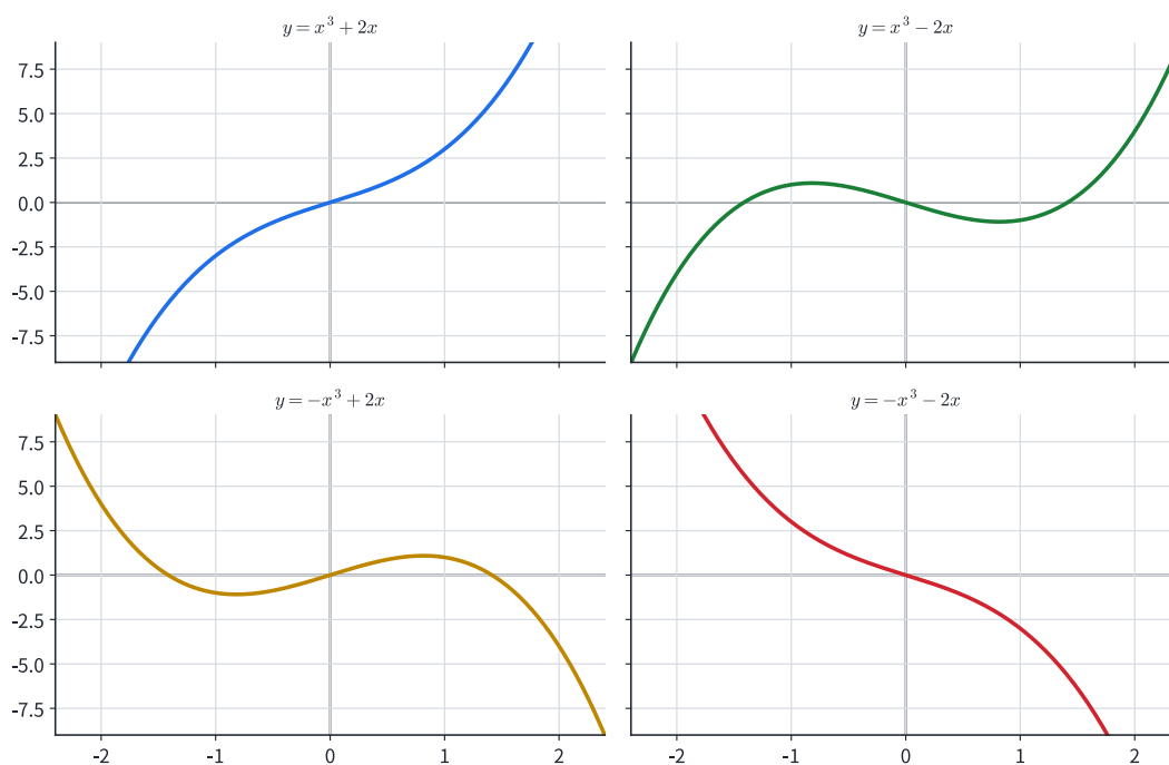
圖 8 | 四組 a, p 皆關於原點點對稱； a 固定兩端， p 影響中心附近的走向。
