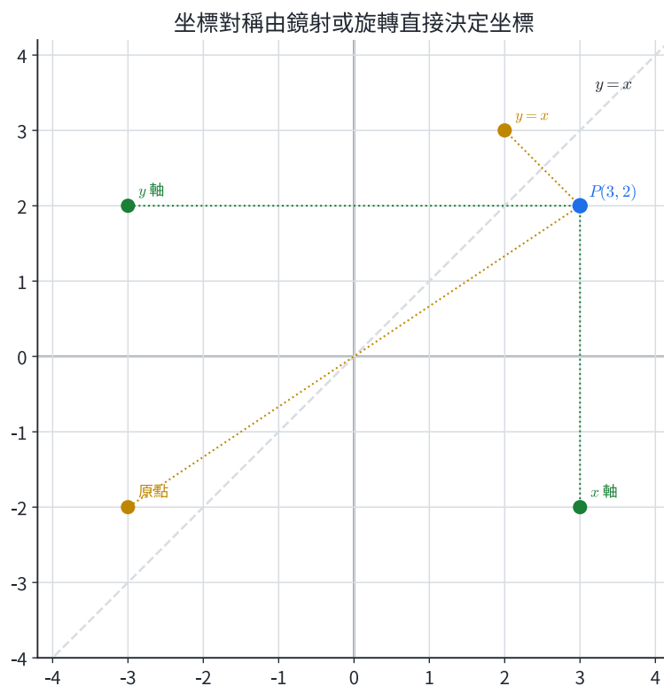
圖 2 | 同一點關於坐標軸、原點與 y = x 的像點；虛線連線對應鏡射或旋轉。
