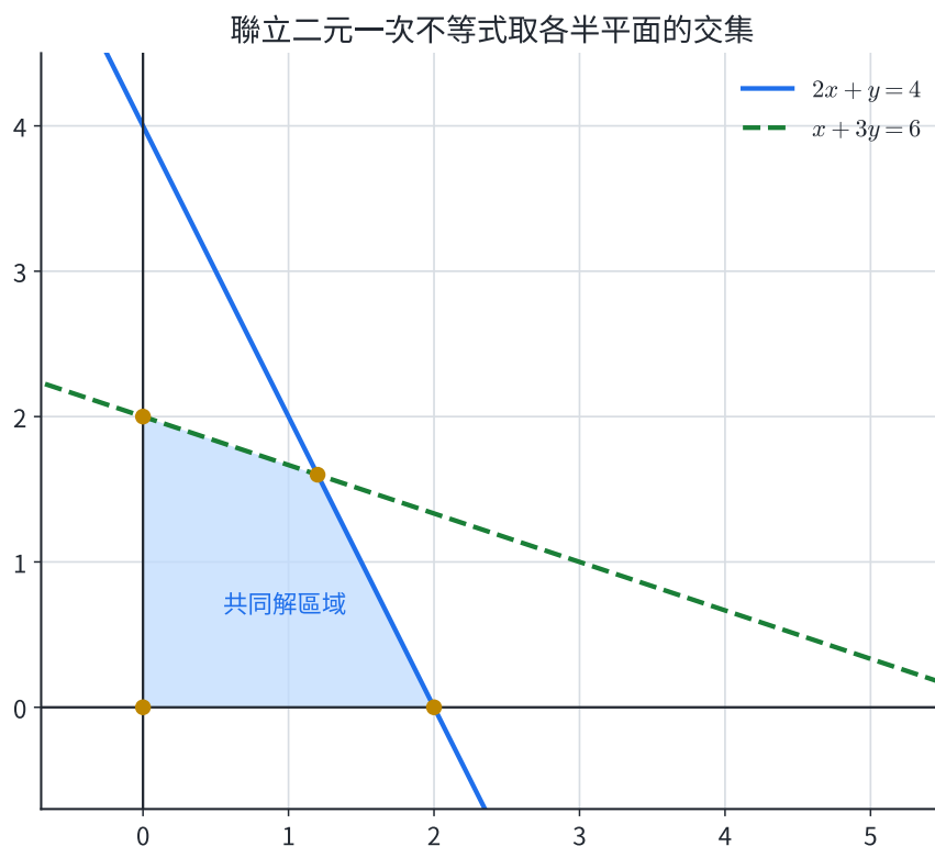
圖 5 | 每個不等式給出一個半平面；共同解是所有半平面的交集。
