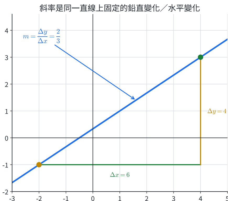
圖 1 | 同一直線上任取兩點，斜率三角形的鉛直變化與水平變化維持固定比例。
