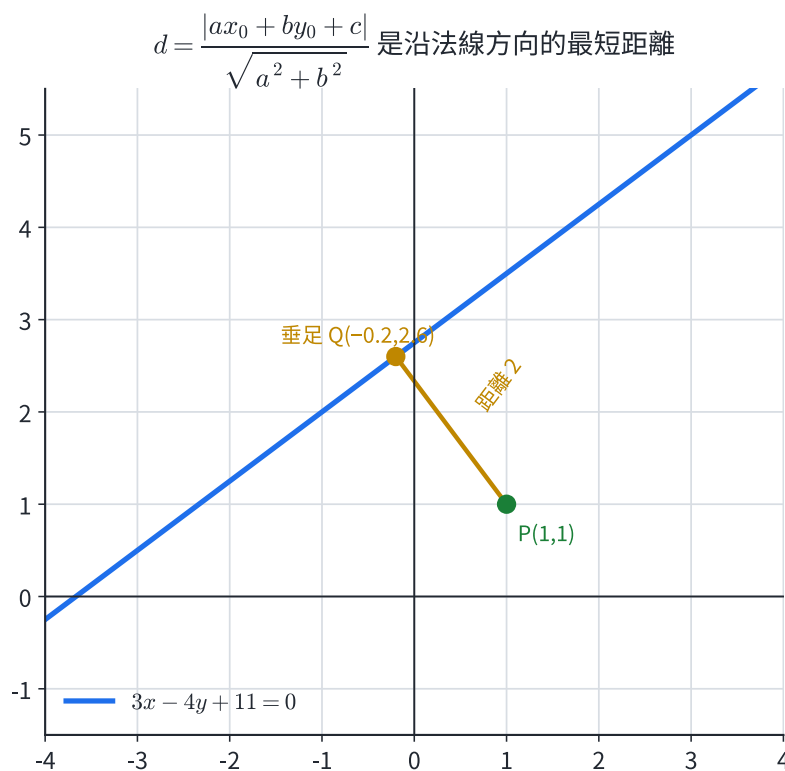
圖 3 | 從點 P 沿直線法向量作垂線，與原直線的交點就是垂足。
