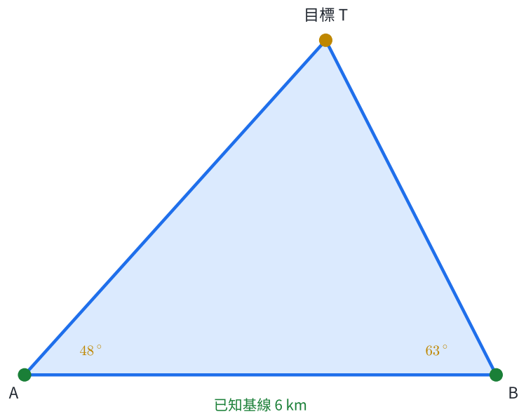
圖 10 | 基線三角測量由一邊兩角定位遠端目標。
