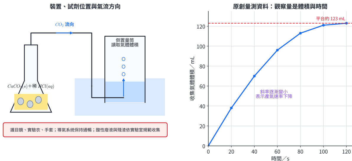
圖 9 | CaCO 3 與稀鹽酸產生 CO 2 的排水集氣裝置及原創體積—時間資料；導管出口位於倒置量筒開口內，氣泡向上進入集氣區。
