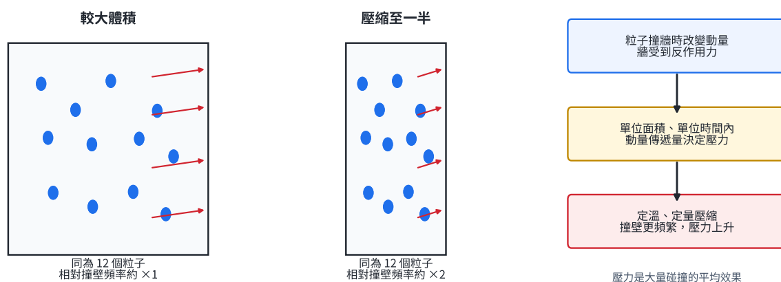
圖 1 | 同數粒子由較大空間壓縮至一半體積後，單位時間撞壁次數增加；紅箭頭標出對同一側器壁的動量傳遞。
