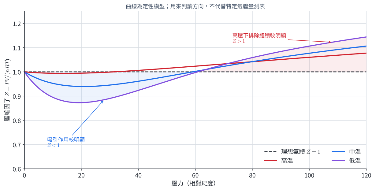
圖 8 | 三條定性 Z -壓力曲線。低溫曲線的吸引作用谷值較深；高壓端三條曲線皆逐漸受到排除體積影響。
