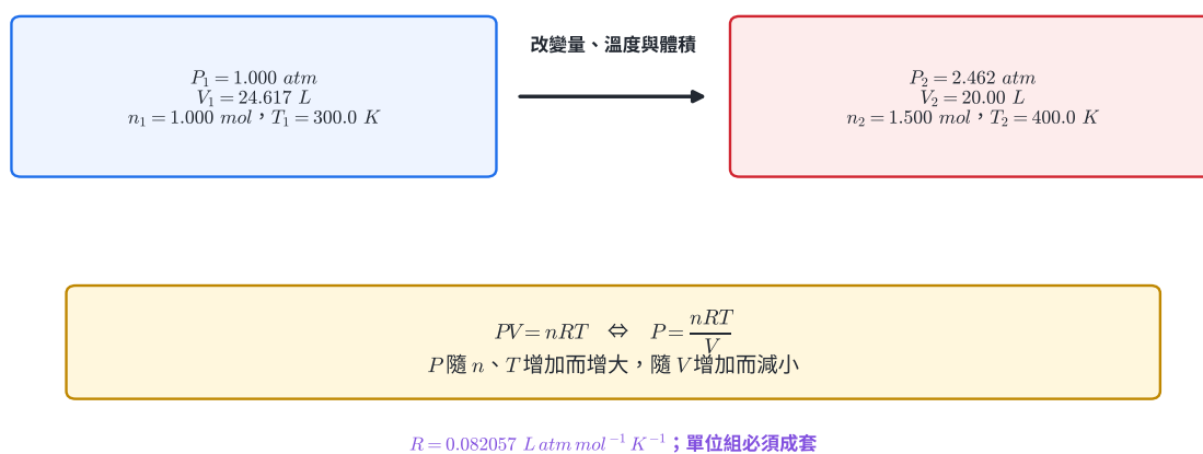
圖 6 | 兩個理想氣體狀態以 PV = nRT 連接；狀態 2 的莫耳數與溫度增加、體積減小，因此壓力上升至 2.462 atm。
