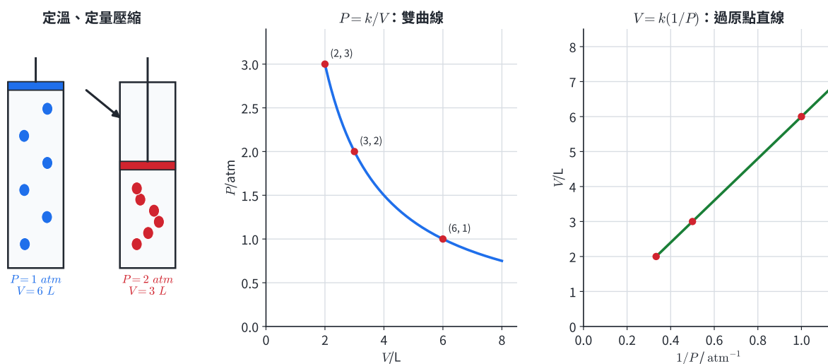
圖 3 | 同一份定溫氣體由 6 L、1 atm 壓縮至 3 L、2 atm； P - V 圖為雙曲線， V - 1/P 圖為過原點直線。
