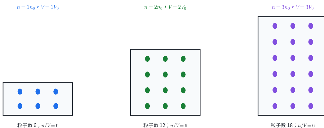
圖 5 | 同溫同壓下，粒子數、莫耳數與容器體積依 1:2:3 同比例增加；每單位體積的粒子數保持相同。
