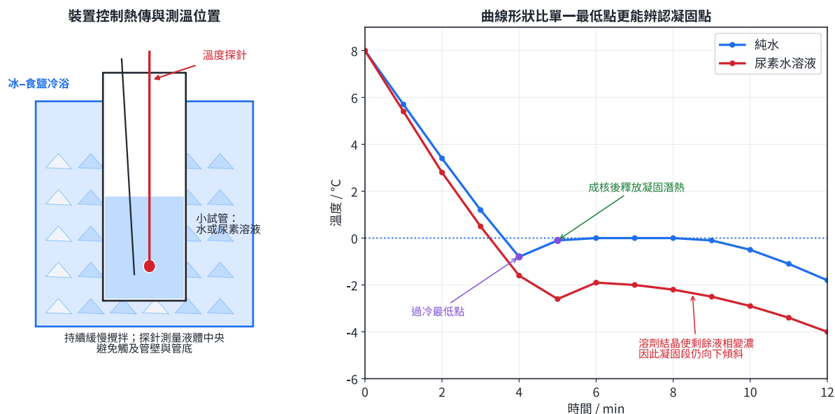
圖 8 | 凝固點實驗的同軸試管、測溫位置與原創冷卻資料；純水有過冷後回升與平臺，溶液在結冰段仍持續降溫。
