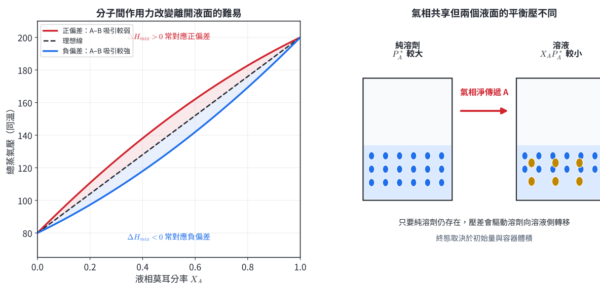
圖 6 | 非理想溶液的正、負蒸氣壓偏差，及密閉容器中純溶劑向較低蒸氣壓溶液的淨轉移。
