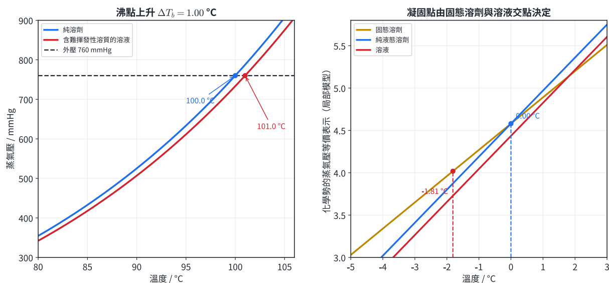
圖 7 | 同一個蒸氣壓下降同時移動沸騰與凝固的交點；沸點向高溫移，凝固點向低溫移。
