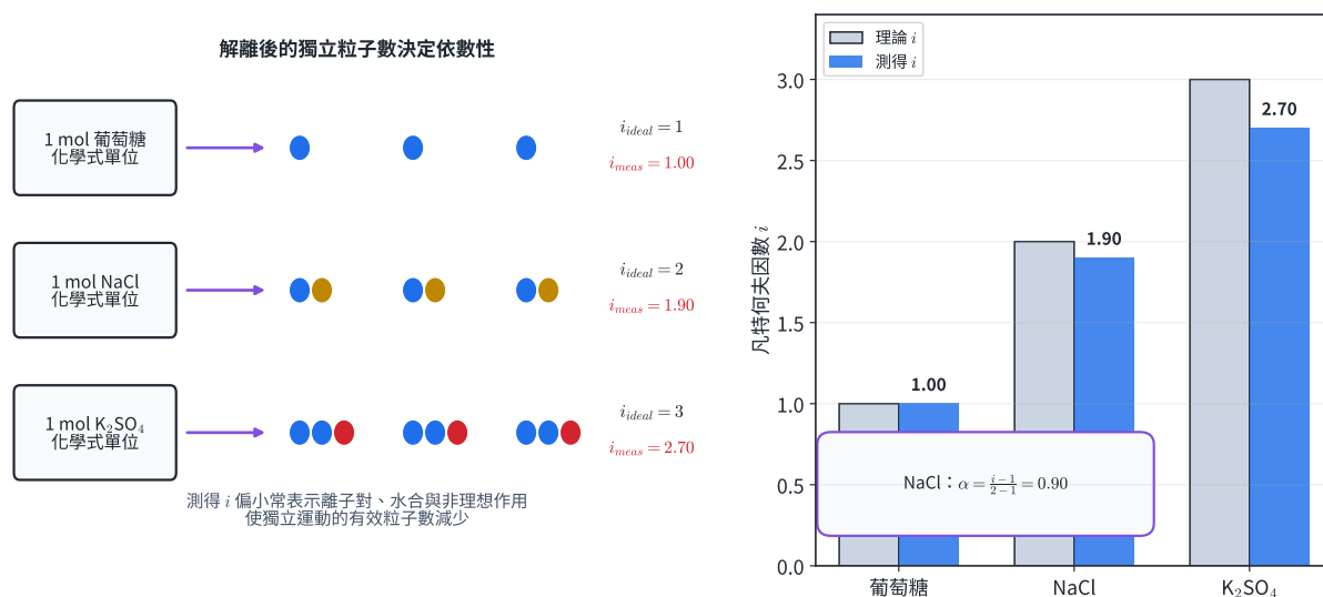
圖 10 | 葡萄糖、NaCl 與 K_2SO_4 的理論粒子帳與一組測得 i ；電解質測得值低於完全解離整數，可用離子對與非理想作用解釋。
