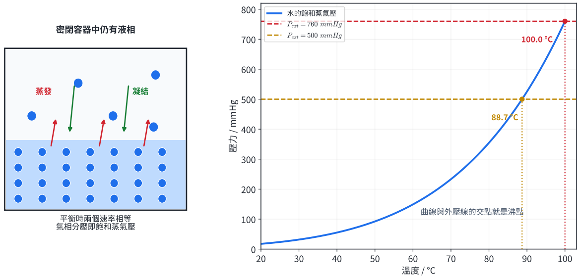
圖 3 | 密閉容器的蒸發-凝結動態平衡，及水的飽和蒸氣壓曲線與 760、500 mmHg 外壓的交點。
