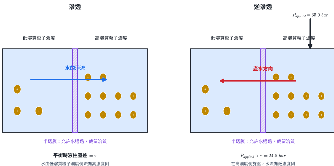
圖 9 | 滲透時水流向較高溶質粒子濃度側；逆滲透在高濃度側施加大於滲透壓的操作壓力，使水的淨流反向。
