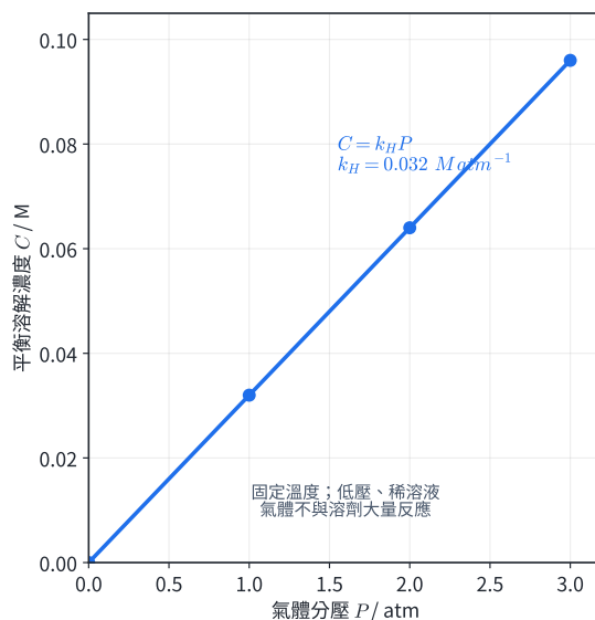
圖 2 | 固定溫度的亨利定律；分壓由 1 atm 增至 3 atm 時，模型中的平衡溶解粒子數與濃度等比增加。
