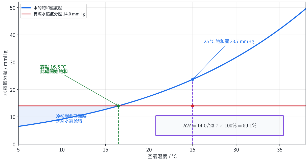
圖 4 | 實際水蒸氣分壓 14.0 mmHg 時，25 °C 的相對濕度由縱向比值得到；橫線與飽和曲線的交點約 16.5 °C，即露點。
