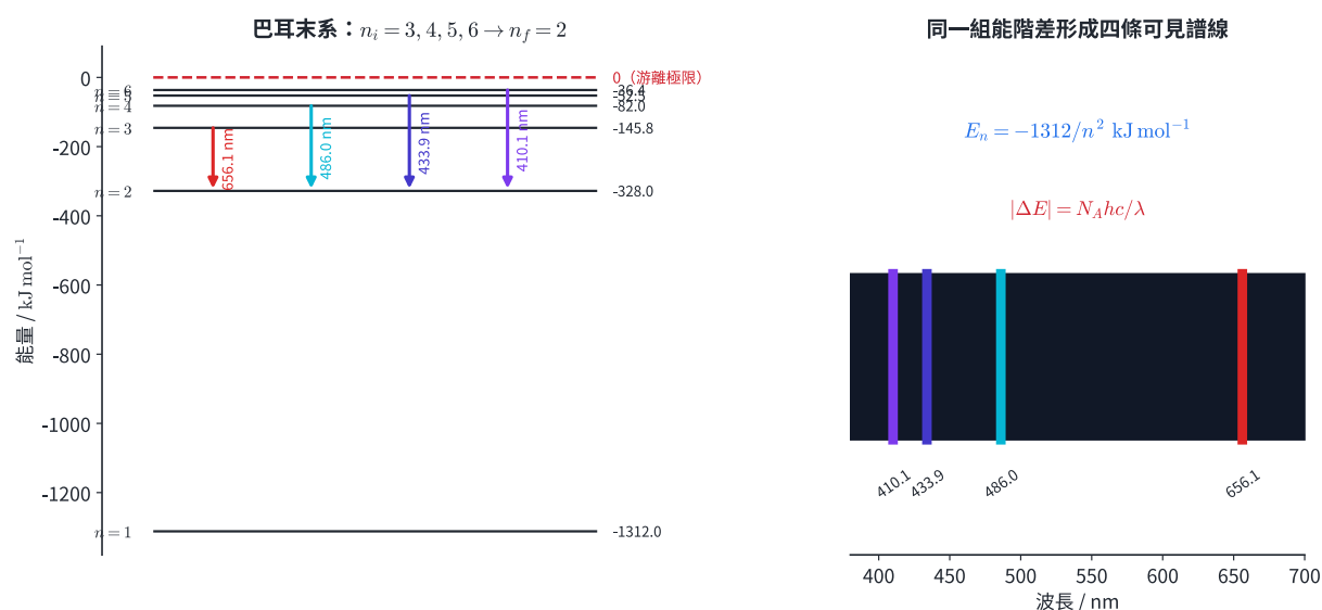
圖 4 | 氫原子能階、巴耳末系四條轉移與相同波長的線光譜。圖中能階位置由 -1312/n^2 計算。
